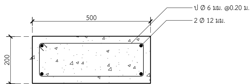
รูปตัด D มาตราส่วน 1:10 *หมายเหตุ หน่วยเป็น มม.
