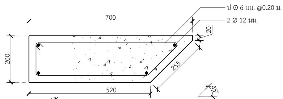
รูปตัด B มาตราส่วน 1:10 *หมายเหตุ หน่วยเป็น มม.
