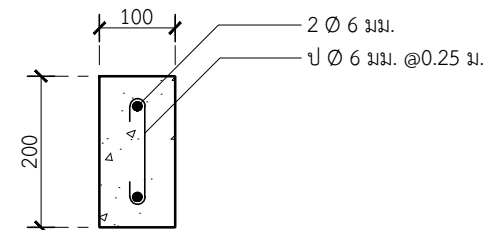
แบบขยายเสาเอ็นกว้าง 20 ซม. มาตราส่วน 1:10
