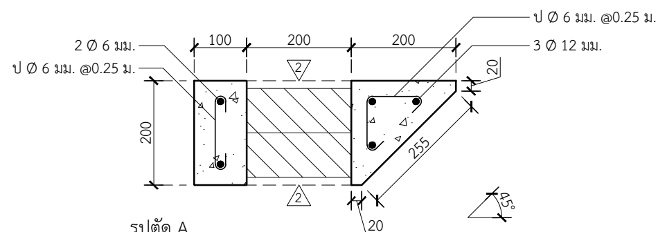
รูปตัด A มาตราส่วน 1:10 *หมายเหตุ หน่วยเป็น มม.
