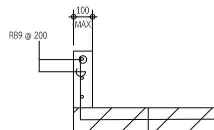
RC. CURB DETAIL SCALE : 1 : 20
