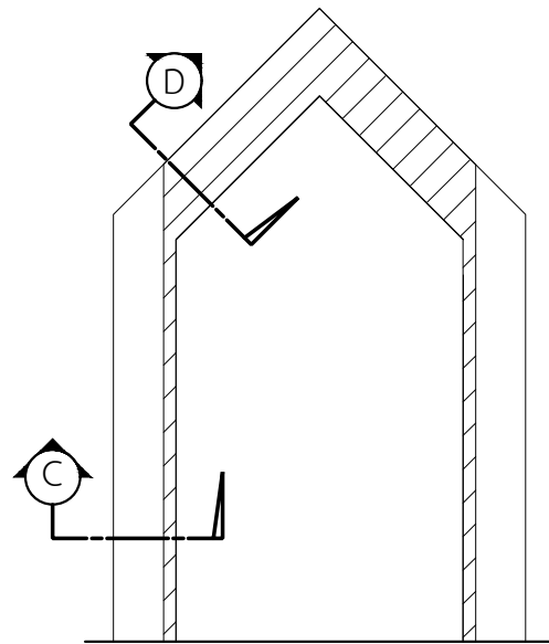
แสดงแนวตัดบัวซุ้มด้านหลัง มาตราส่วน -
