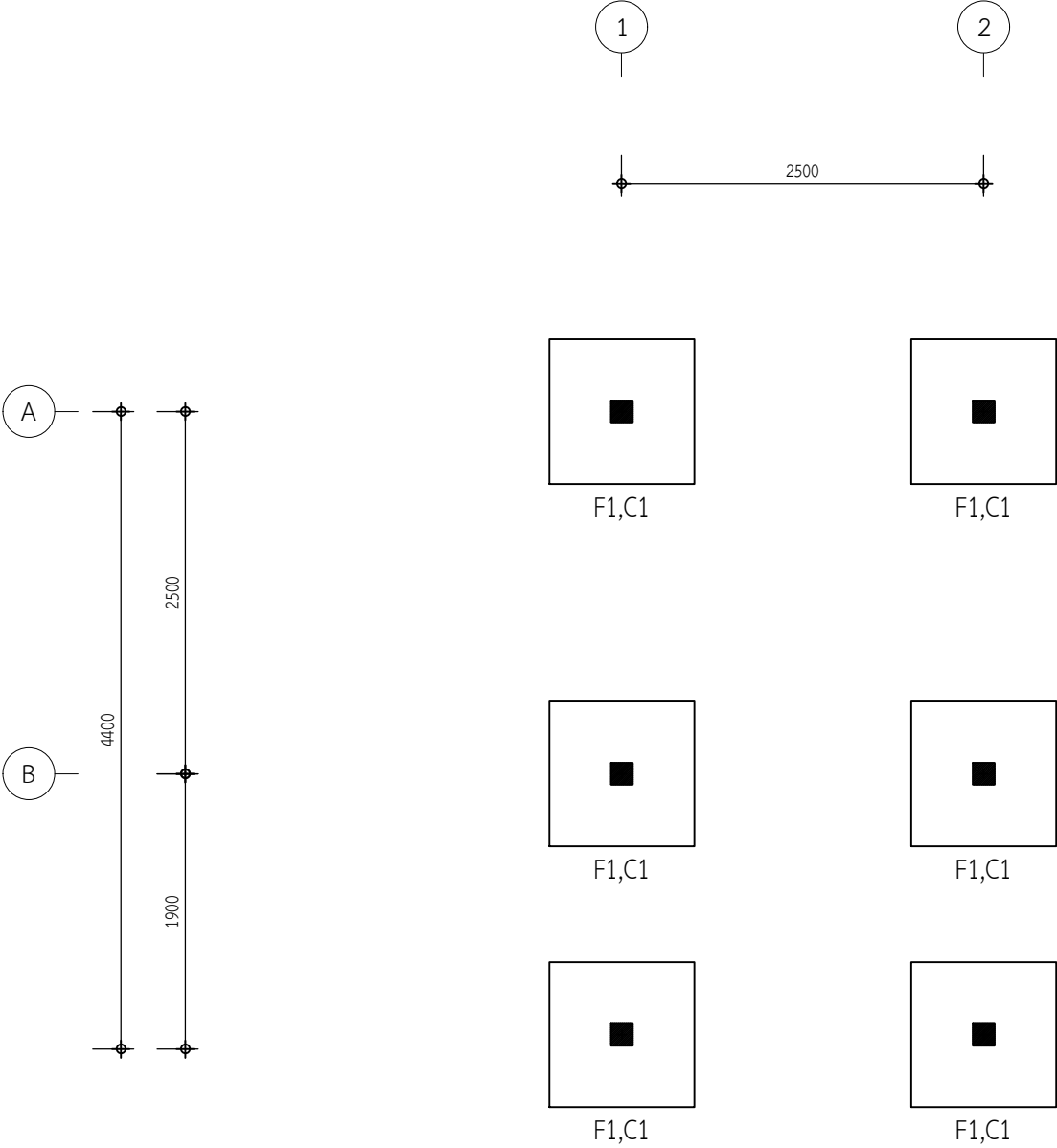
แปลนฐานรากและเสา (กรณีระบบฐานแผ่) SCALE : 1 : 50
