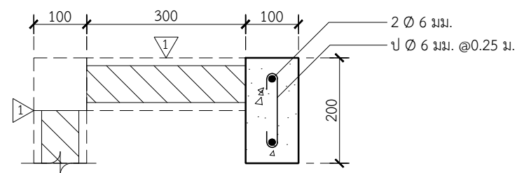
รูปตัด C มาตราส่วน 1:10 *หมายเหตุ หน่วยเป็น มม.
