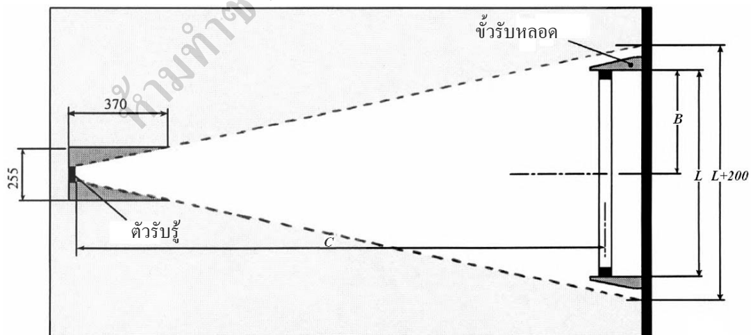
รูปที่ ค.1 มุมมองด้านข้างของระบบการวัดปริมาณแสงออก
