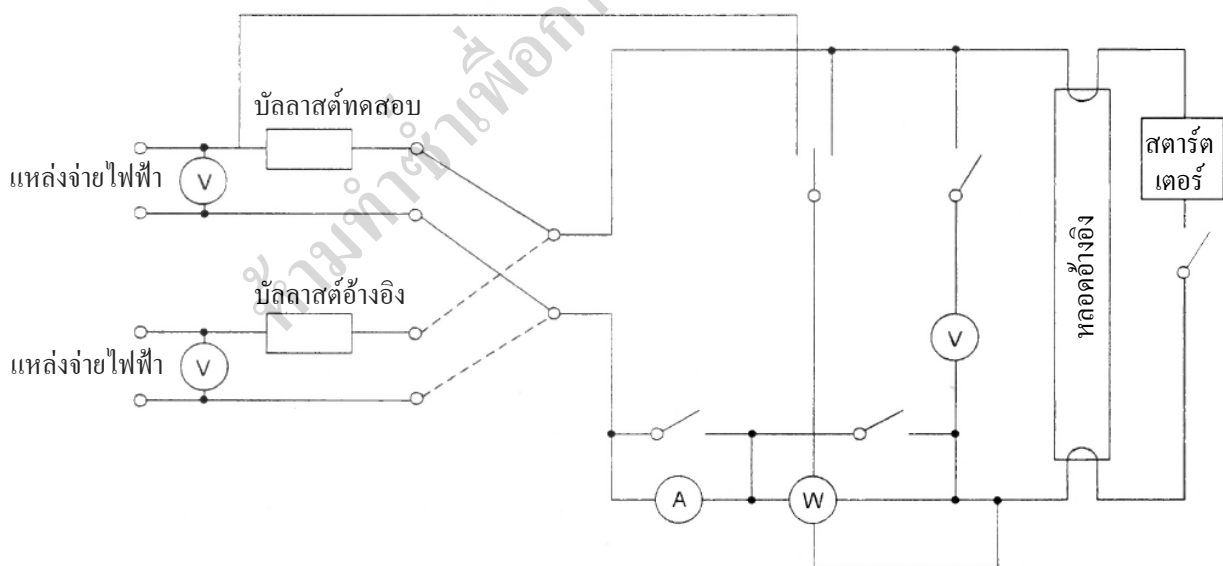
รูปที่ ง.1 ตัวอย่างวงจรบัลลาสต์แกนเหล็ก-หลอด
