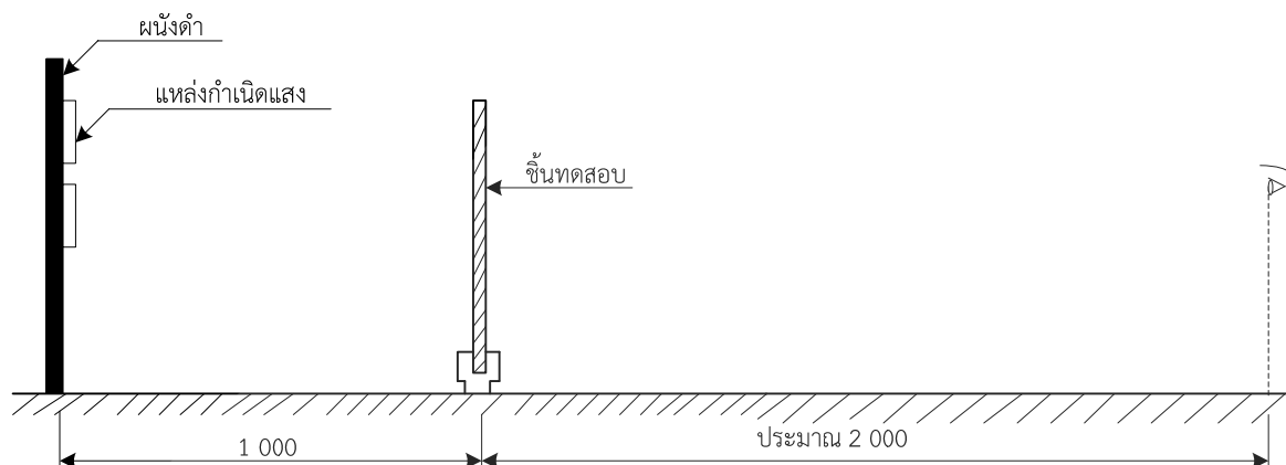
รูปที่ 1 การทดสอบรายการพองอากาศ สิ่งแปลกปลอม ตำแหน่งเป็นจุดรวมเป็นกลุ่ม ตำแหน่งเป็นเส้นหรือเป็นปื้น ต่อเนื่องกัน ตำแหน่งเป็นแนวยาวในเนื้อกระจก ฐาน สนิตปกติ และชุดซีด (ข้อ 9.2.2)
