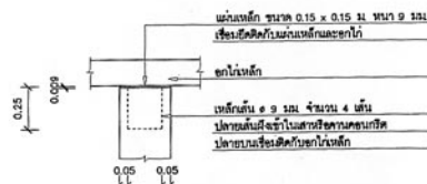
ขยาย ง การติดตั้งคอกไก่เหล็กบนเสาคอนกรีต
