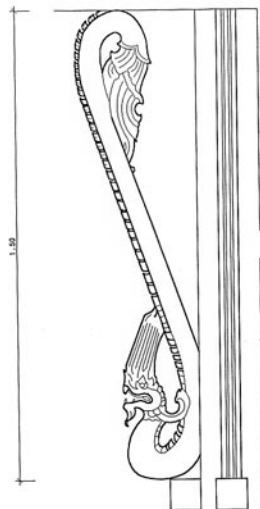
แบบขยายค้ำยัน มาตราส่วน 1 : 10
