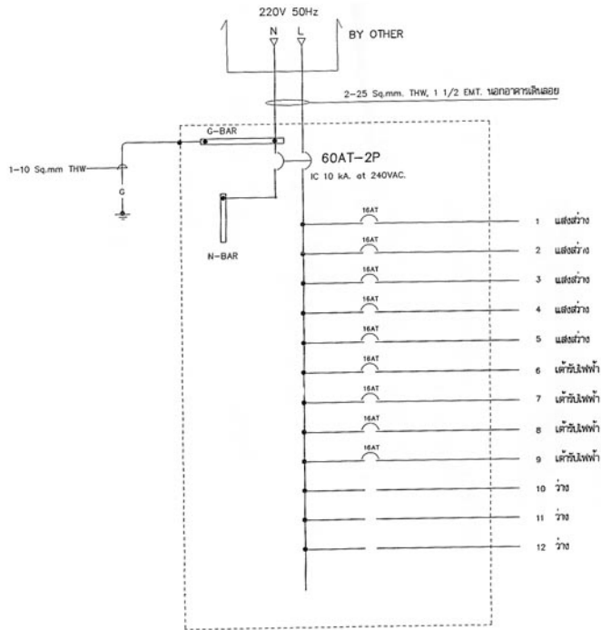
แผนงสวิตซ์อัตโนมัติ " LP "
