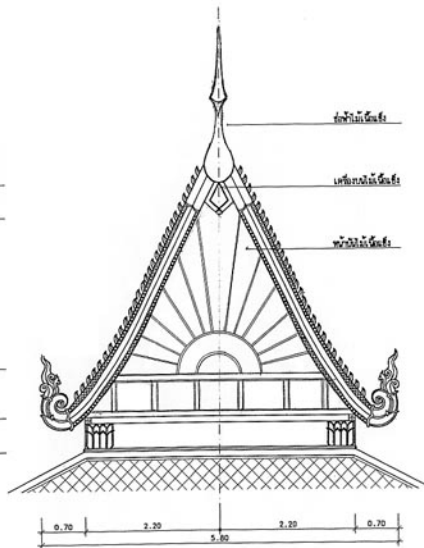
แบบขยายหน้าบัน
