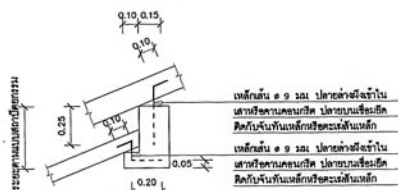
ขยาย ค การตั้งจันทันเหล็กและตะเฒเส้นเหล็กบนเสาหรือคานคอนกรีต RB2
