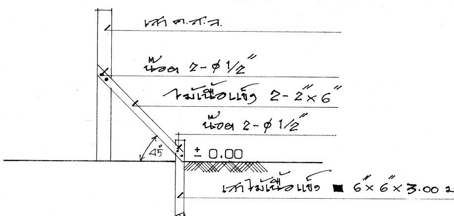
เสายึดกันลัม 1 : 50
