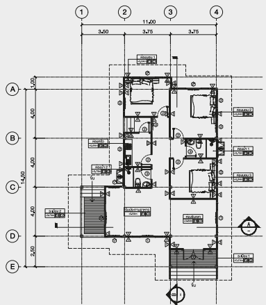
แปลนพื้นที่
