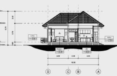
รูปตัด B-B
