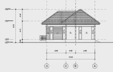
รูปด้าน 2
