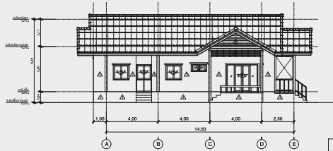
รูปด้าน 4
