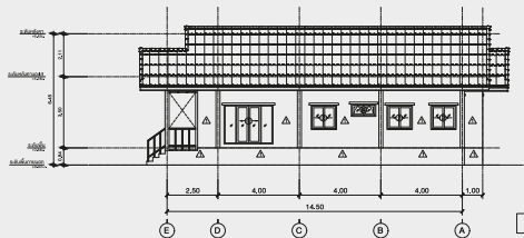
รูปด้าน 2
