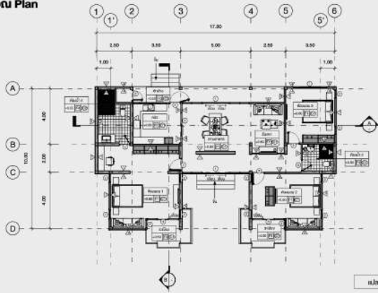
แปลนพื้นที่
