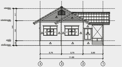
รูปด้าน 3
