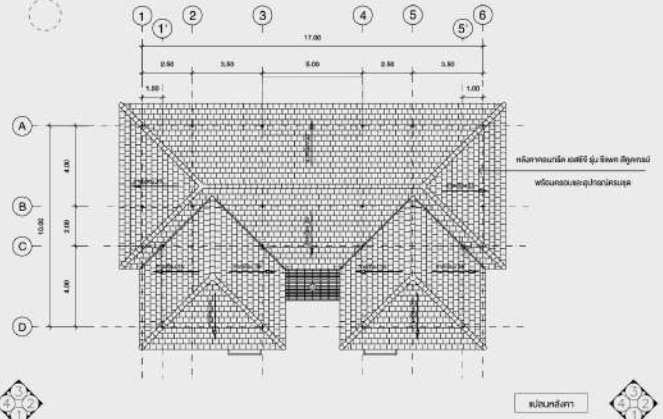
แปลนอาคาร
