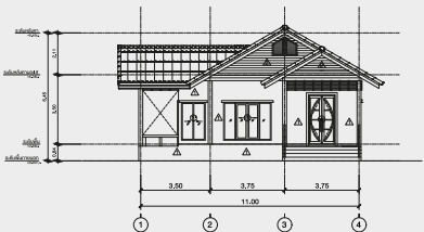
รูปด้าน 1
