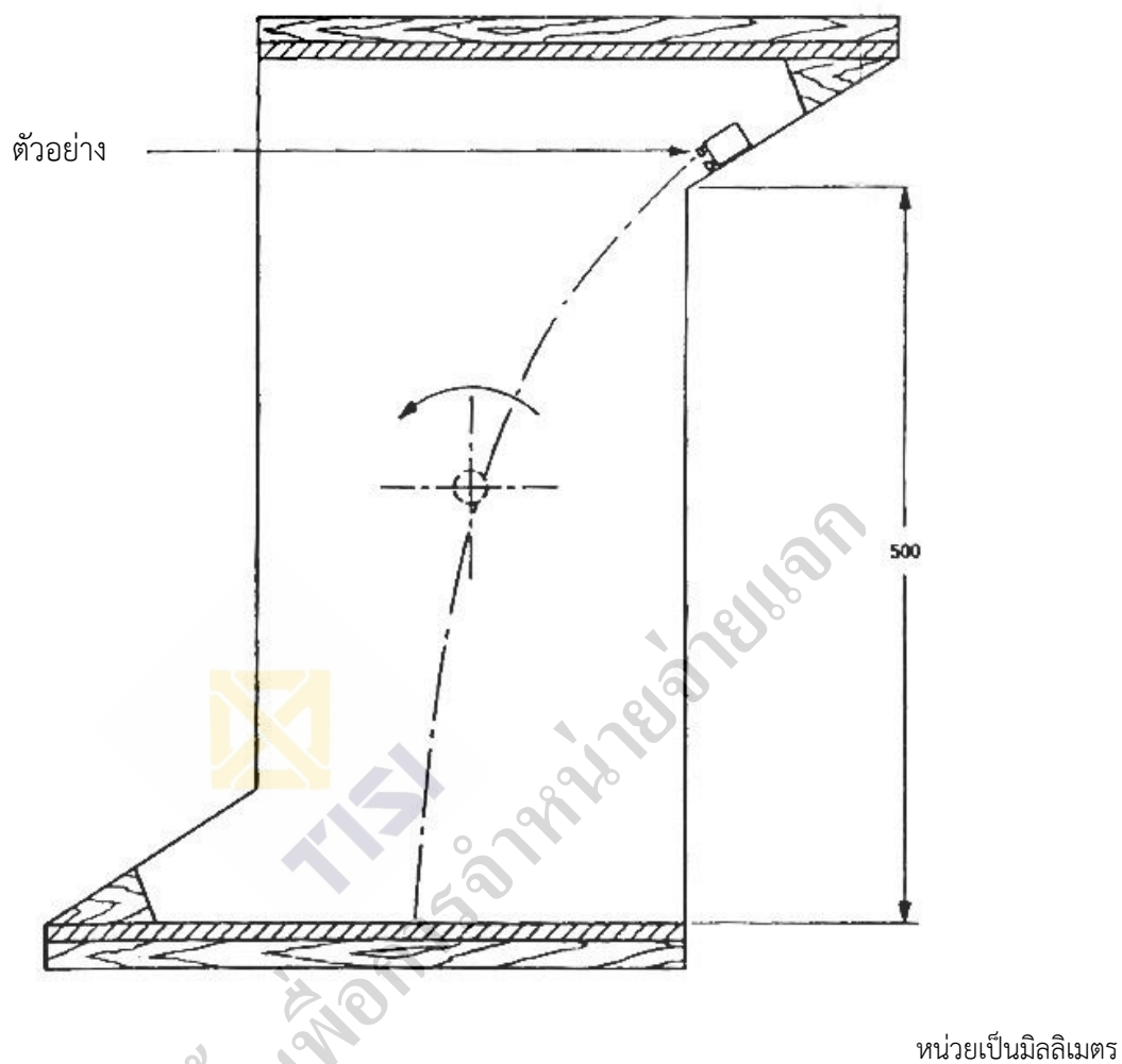
รูปที่ 2 ทัมบลิ้งบาร์เรล
