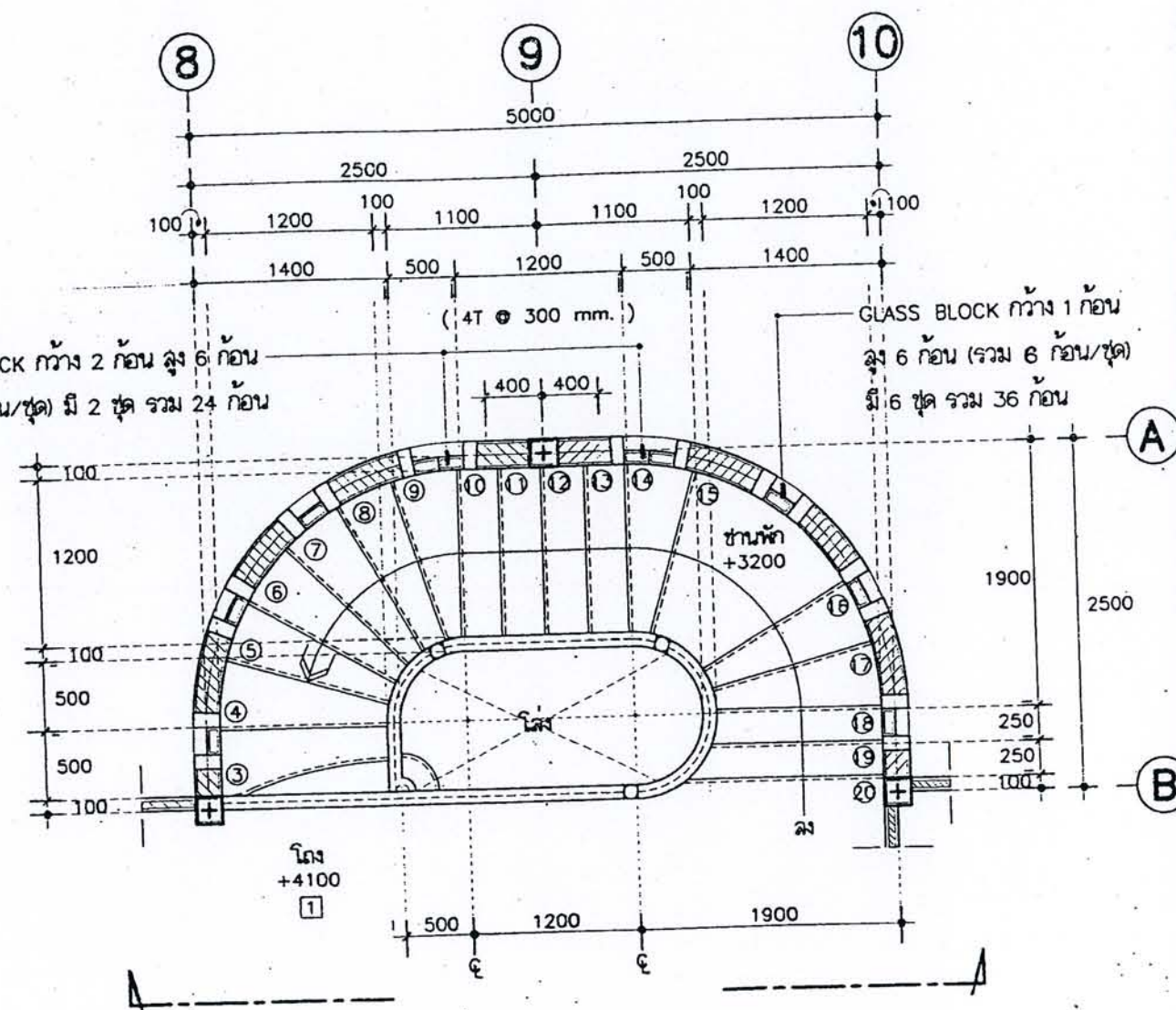
แปลนขยายบ้านโดชั้นบน มาตราส่วน 1 : 50
