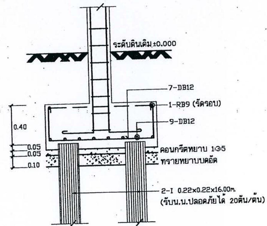
SECTION F2A 1:20
