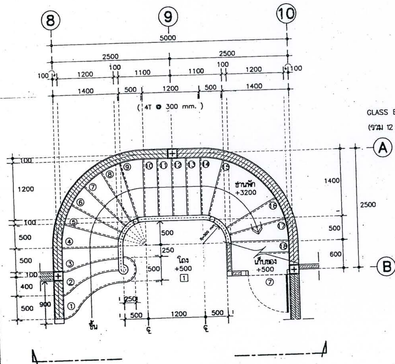
แปลนขยายบ้านโดชั้นล่าง มาตราส่วน 1 : 50
