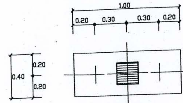
PLAN F2A
