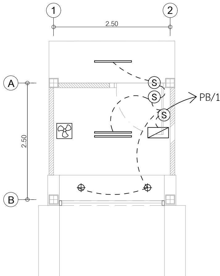
ผังไฟฟ้าแสงสว่าง
