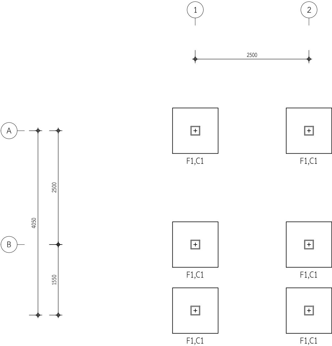
แปลนฐานรากและเสา (กรณีระบบฐานแผ่) SCALE : 1 : 50
