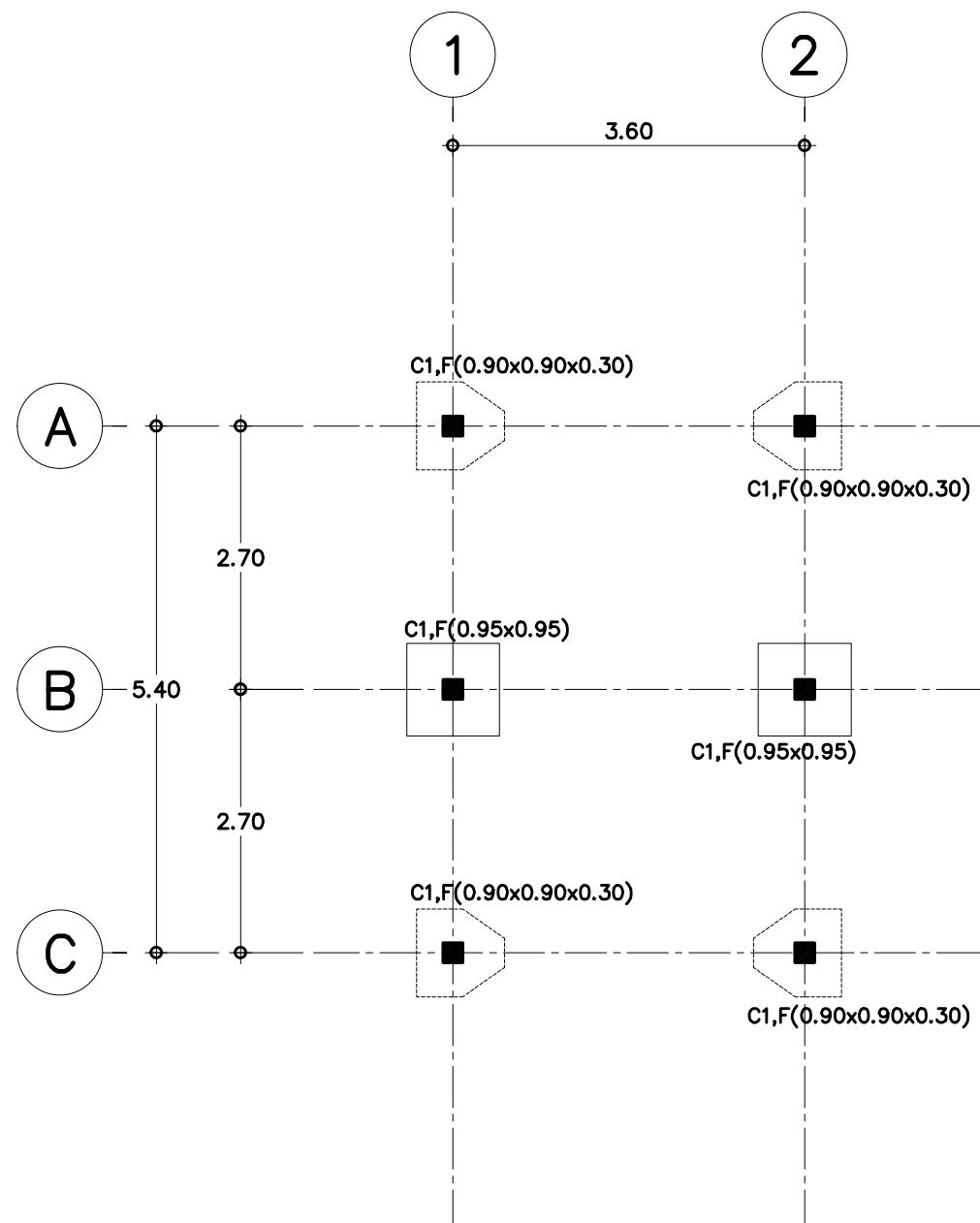
แปลนฐานรากแผ่น , เสาตอม่อ มาตราส่วน 1: 75
