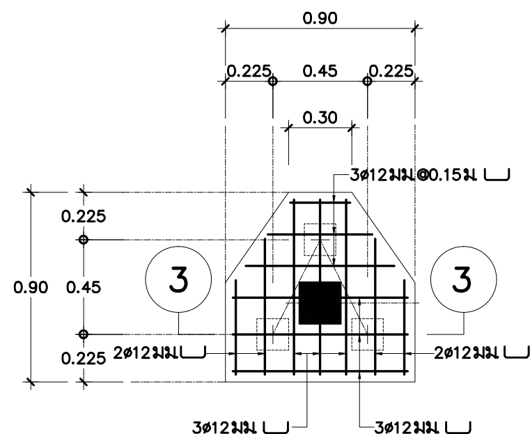
แปลนแสดงการเสริมเหล็ก มาตราส่วน 1: 25
