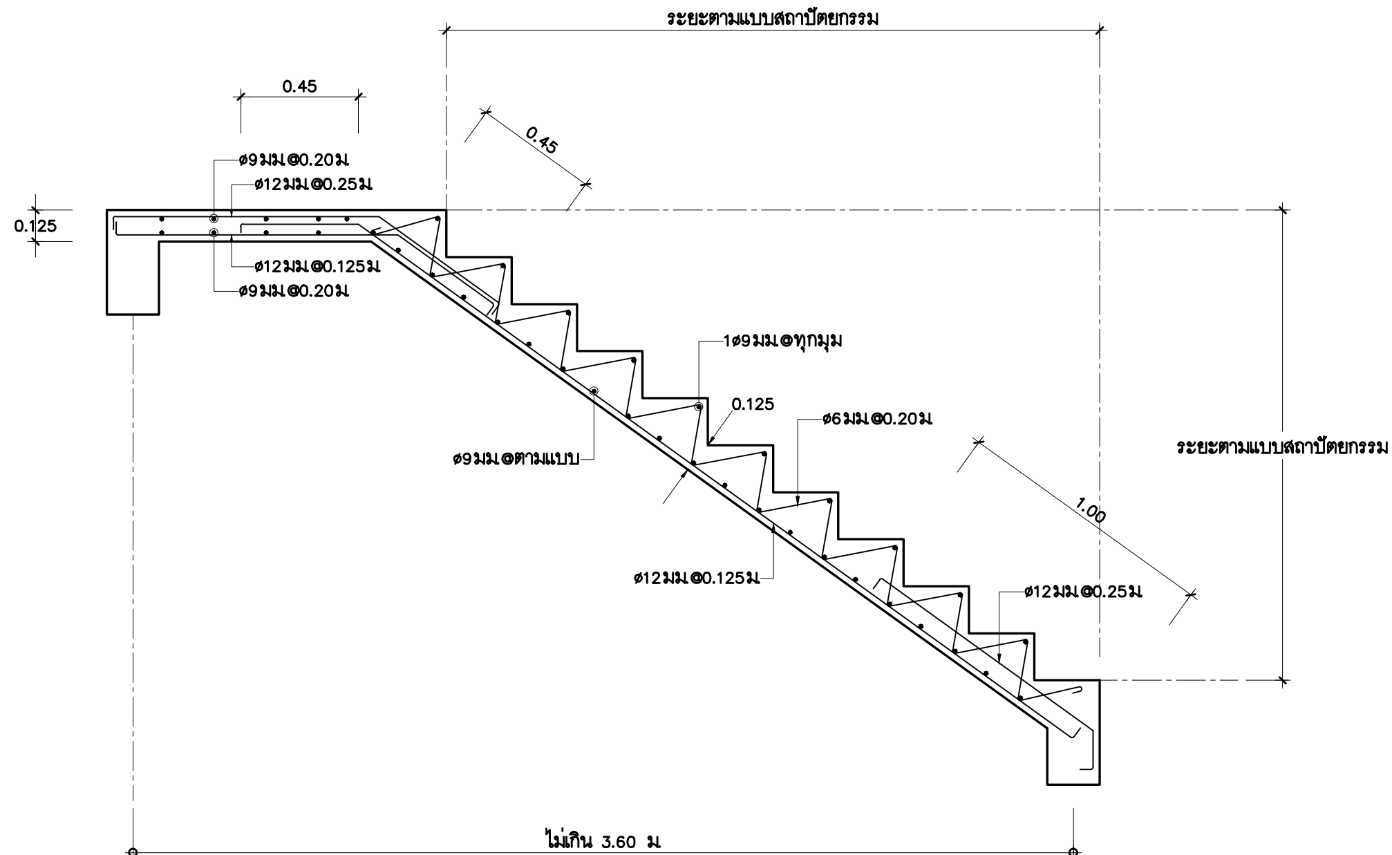
ST1 มาตราส่วน 1:20
