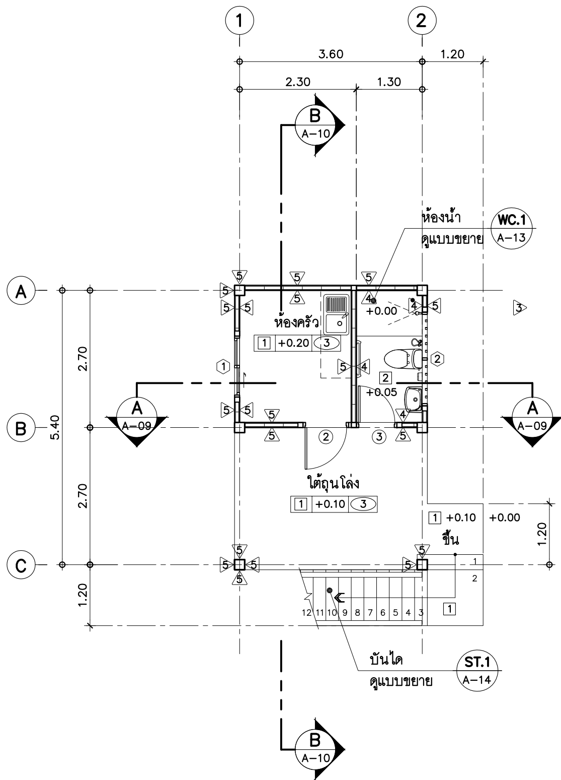
แปลนพื้นที่ชั้นล่าง มาตราส่วน 1 : 75
