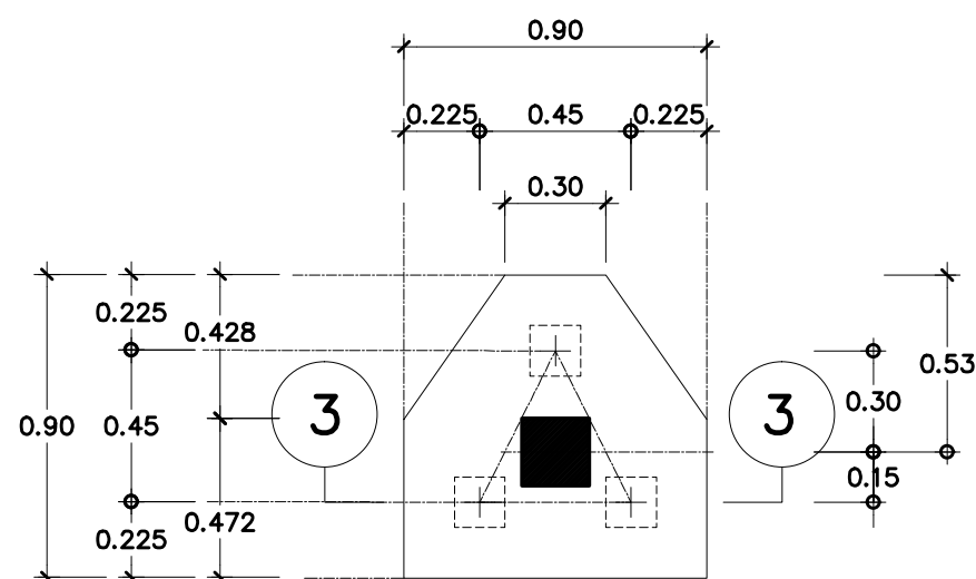
F3 มาตราส่วน 1: 25
