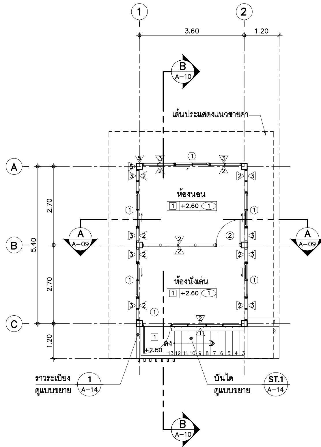
แปลนพื้นที่ชั้นบน มาตราส่วน 1 : 75
