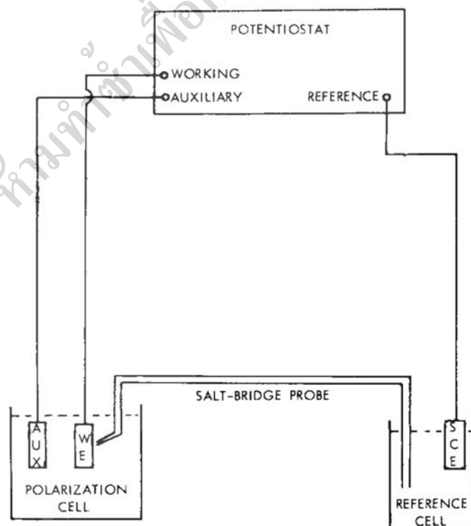
รูปที่ 2-2 แสดงการเตรียมเครื่องโพเทนชิออสเตท และติดตั้งเซลล์ทดสอบ (ข้อ 9.6.4.5)
