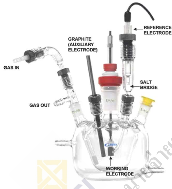
รูปที่ 2-1 แสดงการเตรียมเซลล์ทดสอบ (ข้อ 9.6.4.1)
