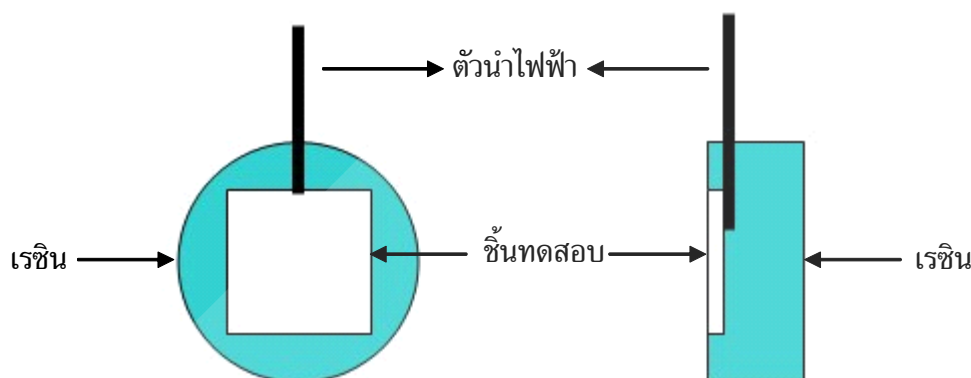
รูปที่ 1 แสดงการติดตัวนำไฟฟ้าและขั้วเรซินขั้วทดสอบ (ข้อ 9.6.3.2)
