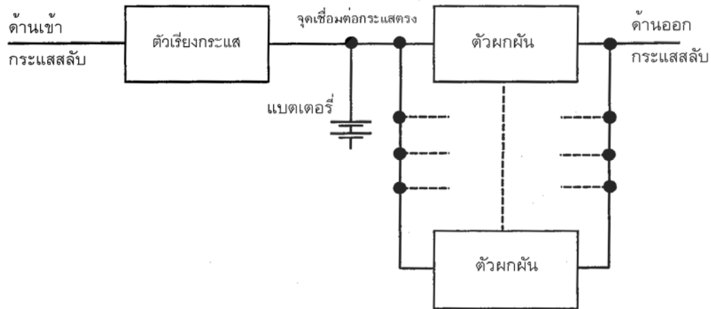
รูปที่ ก.5ก) ยูพีเอสขนานบางส่วน (ที่มีตัวผกผันขนาน) (ข้อ ก.2.1)
