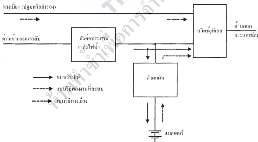
รูปที่ ข.4 การทำงานปฏิสัมพันธ์กับสายของยูฟิเอสที่มีทางเบี่ยง
