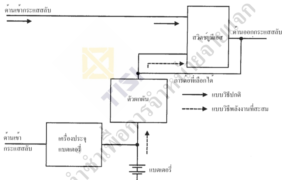
รูปที่ ข.5 การทำงานสำรองสถานะของยูพีเอส
