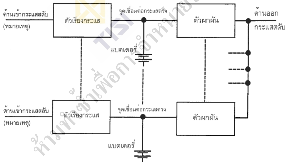
รูปที่ ก.5ข) ยูพีเอสขนาน (ที่มีหน่วยยูพีเอสขนาน) (ข้อ ก.2.1)
