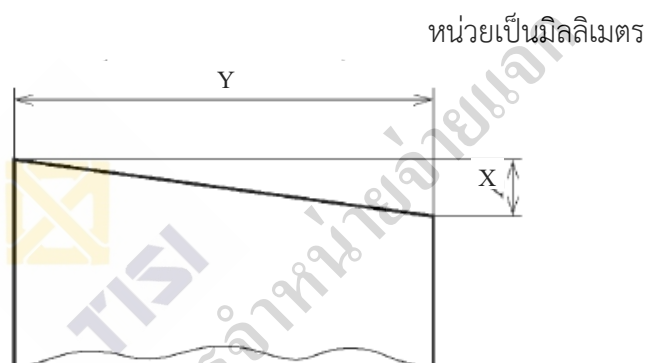
รูปที่ ค.1 การวัดความไม่ตรงฉากแบบตั้งฉาก
