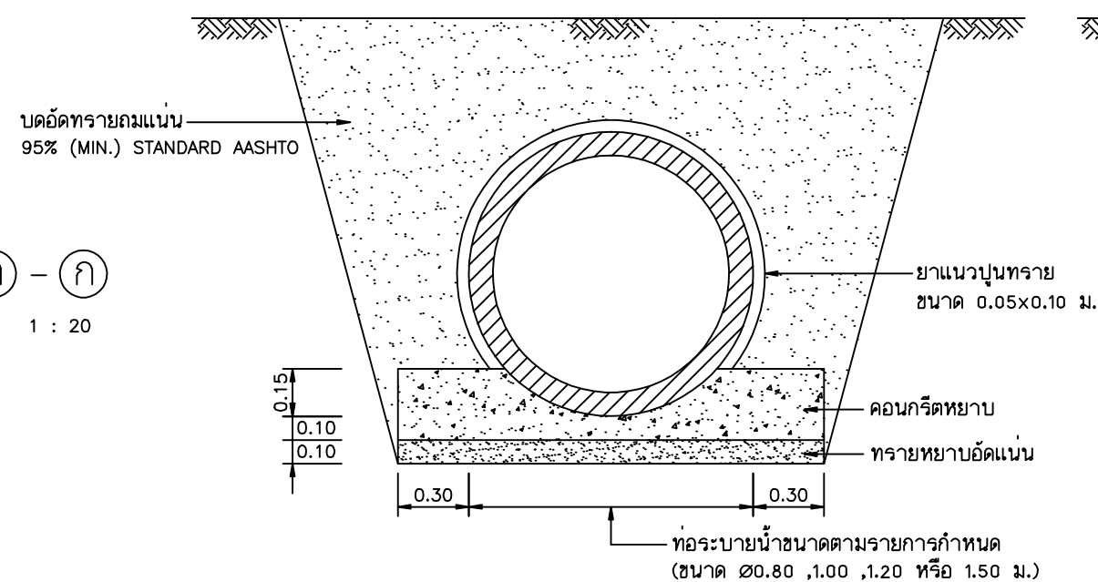
รูปตัดตามขวางท่อระบายน้ำ (ค) - (ค) มาตราส่วน 1 : 20
