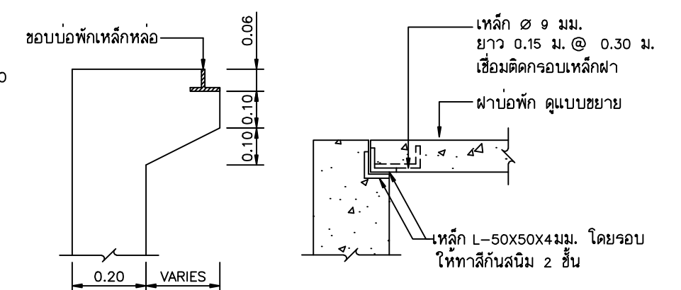
แบบขยาย 2 มาตราส่วน 1 : 10
