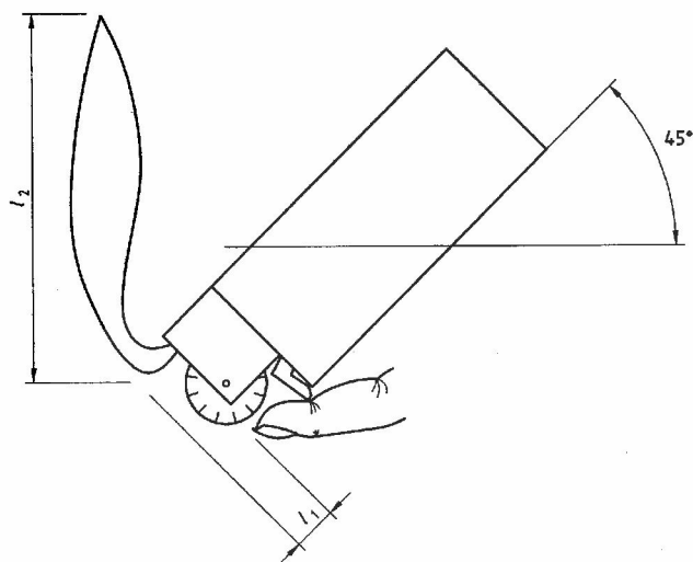
รูปที่ 4 การทดสอบความไม่สม่ำเสมอของเปลวไฟ
