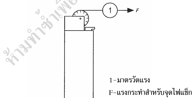
รูปที่ 3 การทดสอบการทำให้เกิดเปลวไฟสำหรับไฟแช็กแบบวงล้อตะไบขีดกับหินขีดไฟ (ข้อ 8.2.1)
