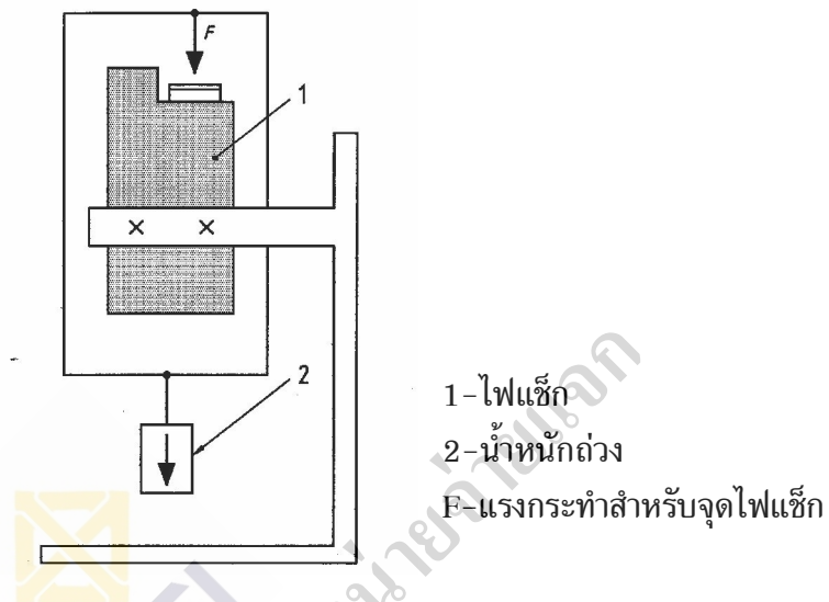
รูปที่ 2 การทดสอบการทำให้เกิดเปลวไฟสำหรับไฟแช็กแบบแม็กเนโต (ข้อ 8.2.1)
