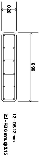
เหล็กเสริมเสาตอนล่าง scale 1 : 20
