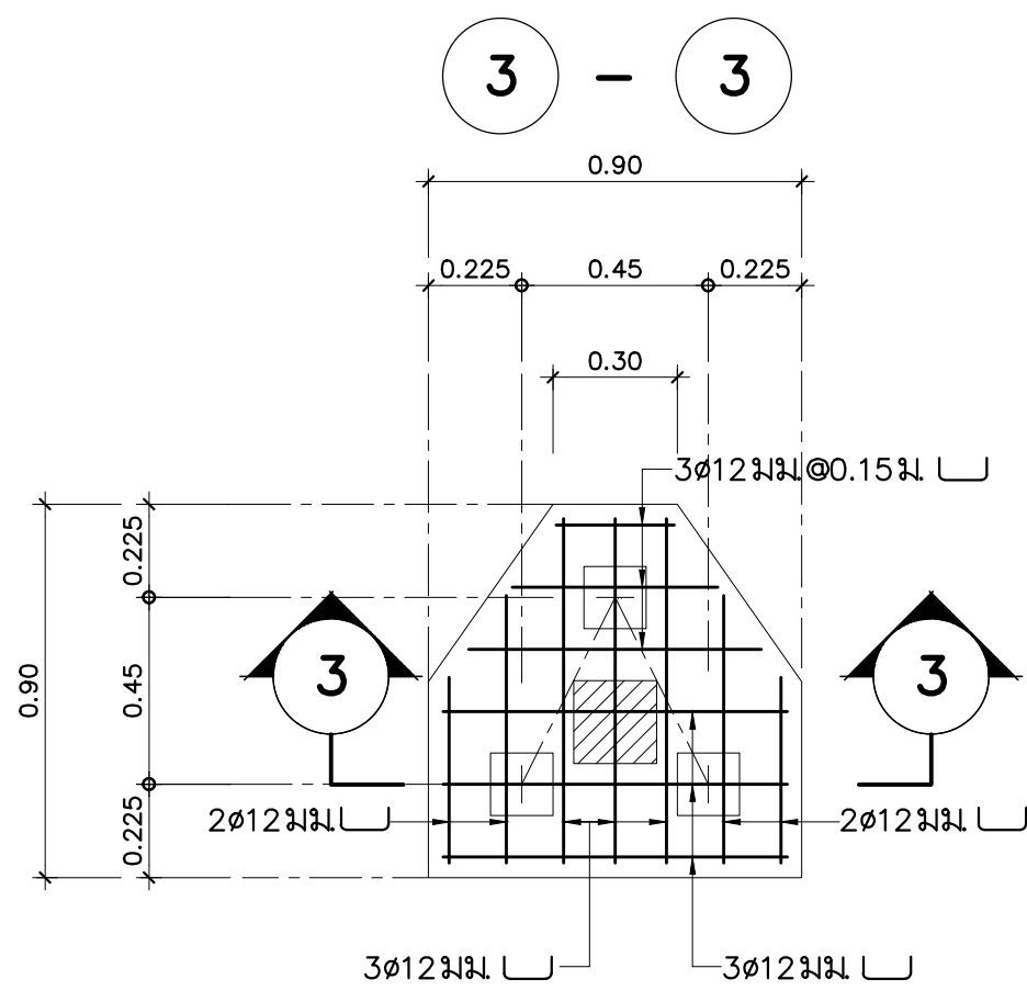
แปลนแสดงการเสริมเหล็ก มาตราส่วน 1 : 20
