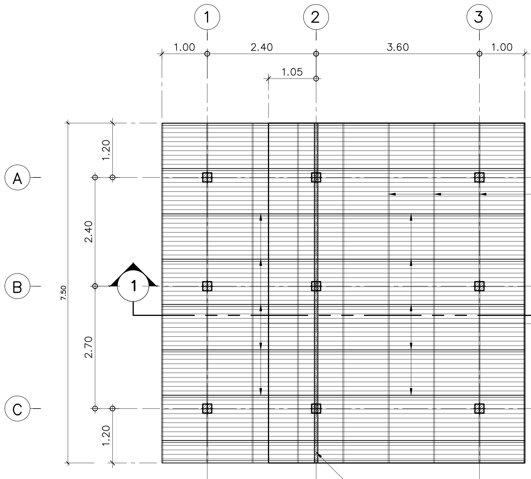
แปลนโครงหลังคา มาตราส่วน 1 : 50
