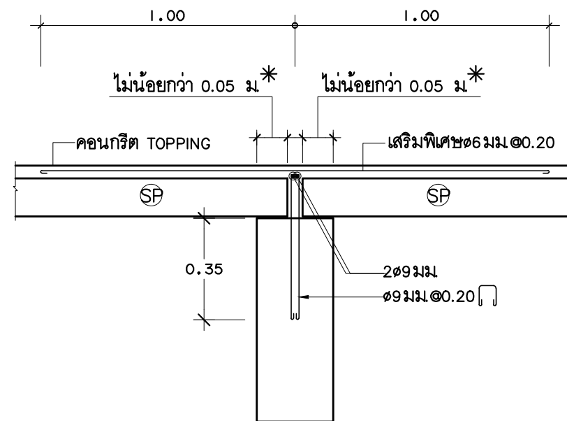
ลักษณะการวางพื้น SP ภายใน
