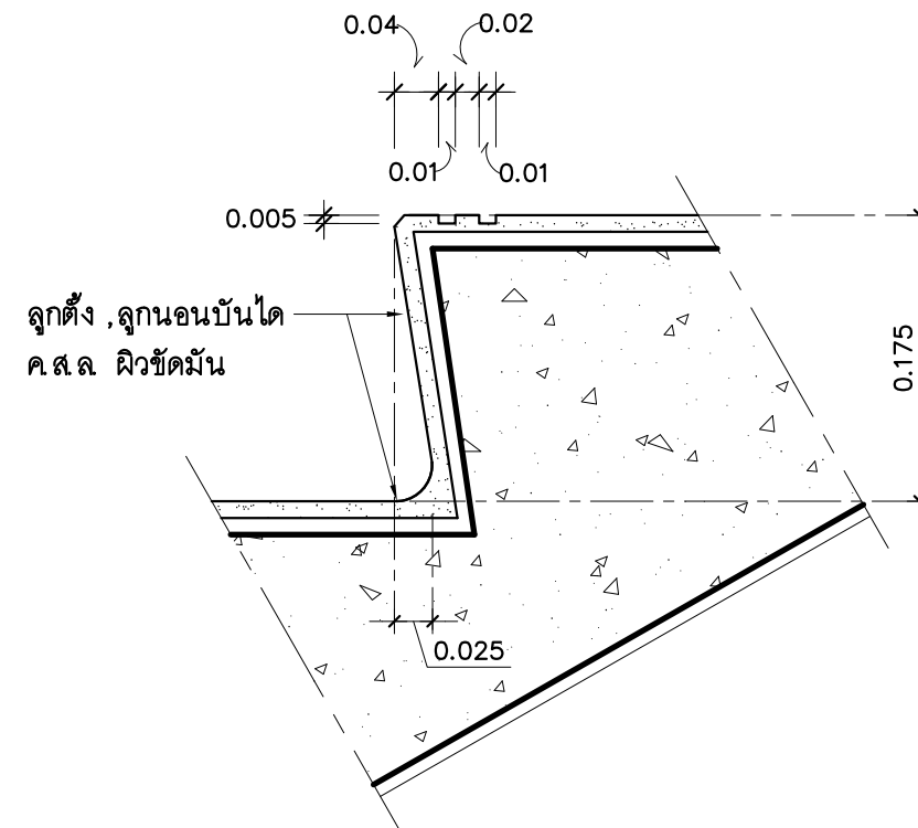
แบบขยายจุมุกบันได มาตราส่วน 1 : 5
