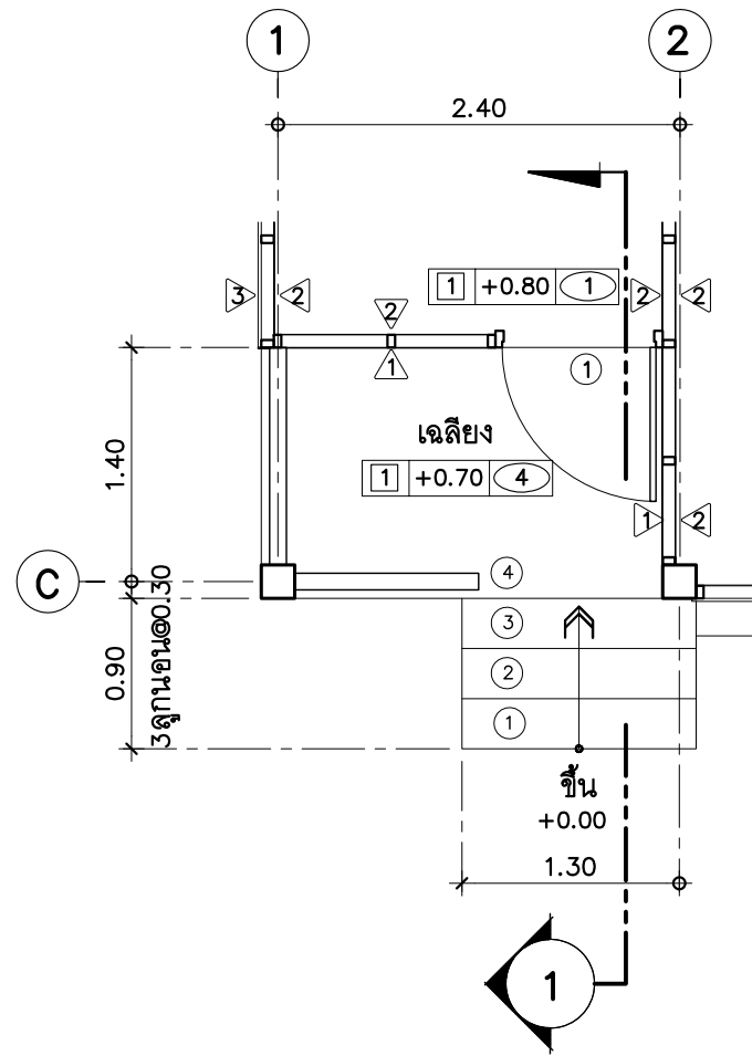
แบบขยายบันได ST.1 มาตราส่วน 1 : 50
