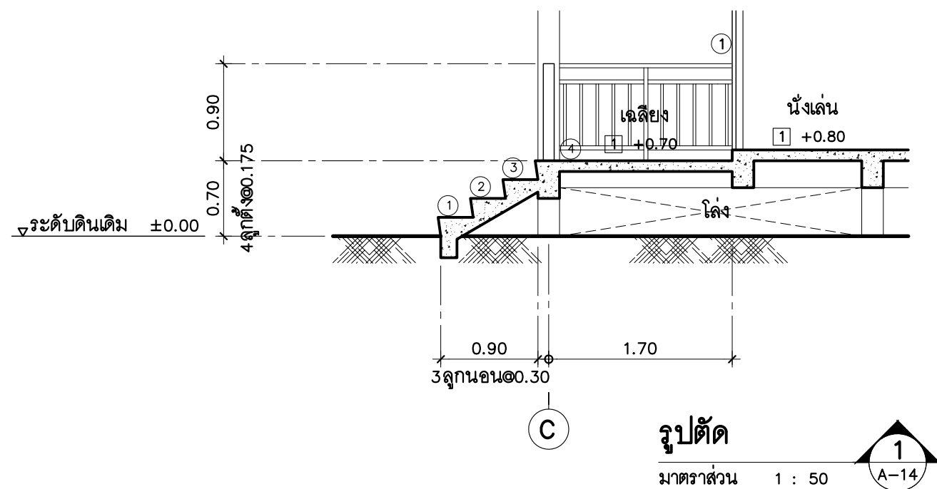
แบบขยายบันได ST.1 มาตราส่วน 1 : 50
