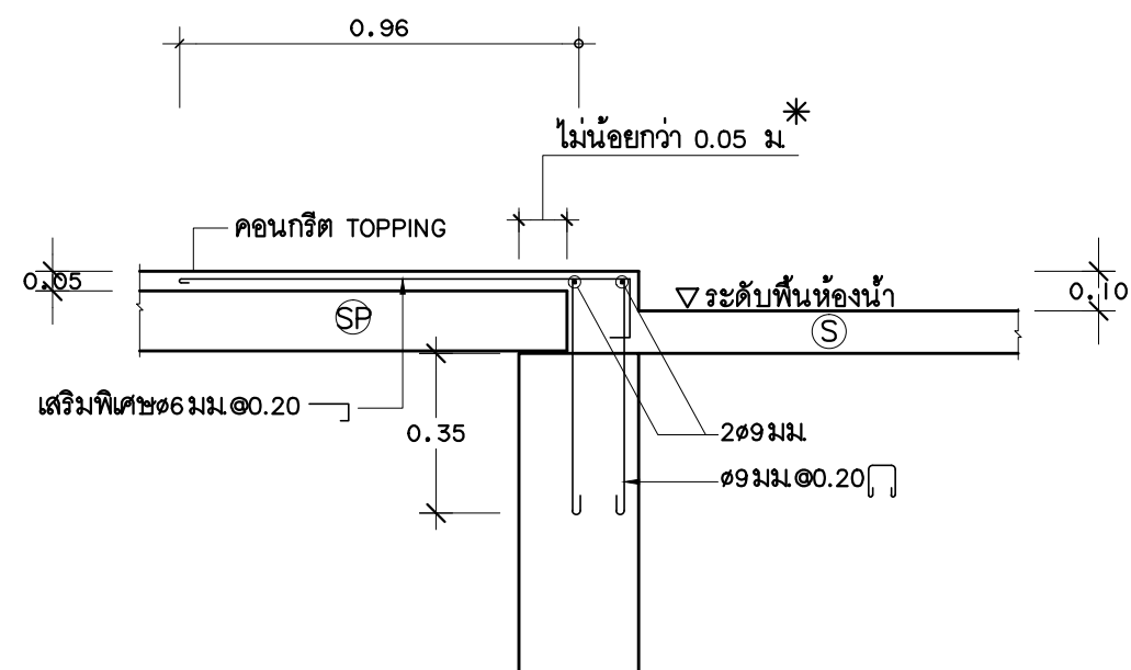
ลักษณะการวางพื้น SP บริเวณพื้นห้องน้ำ
