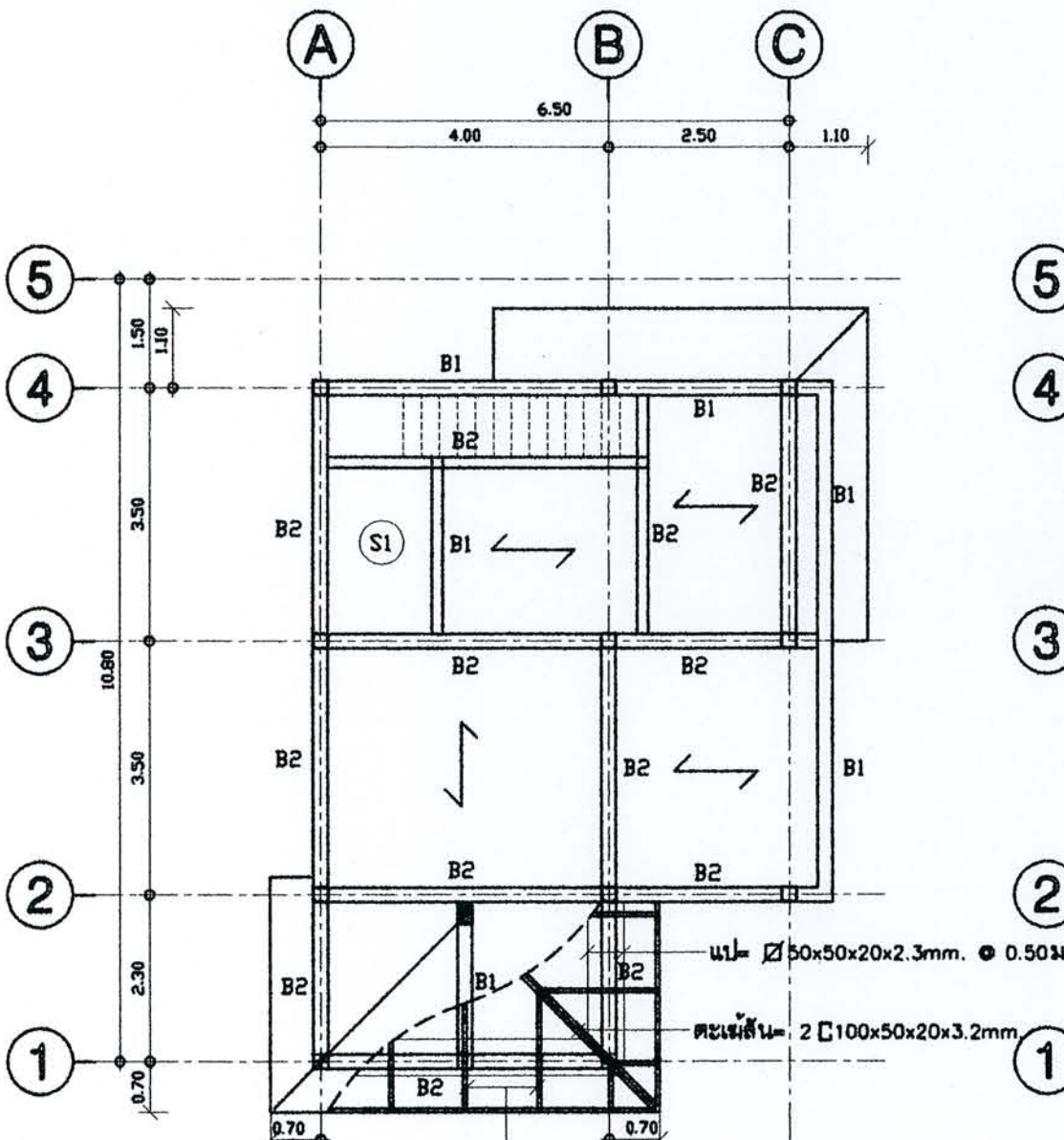
ผังคานพื้นชั้นที่ 2 มาตราส่วน 1:100
