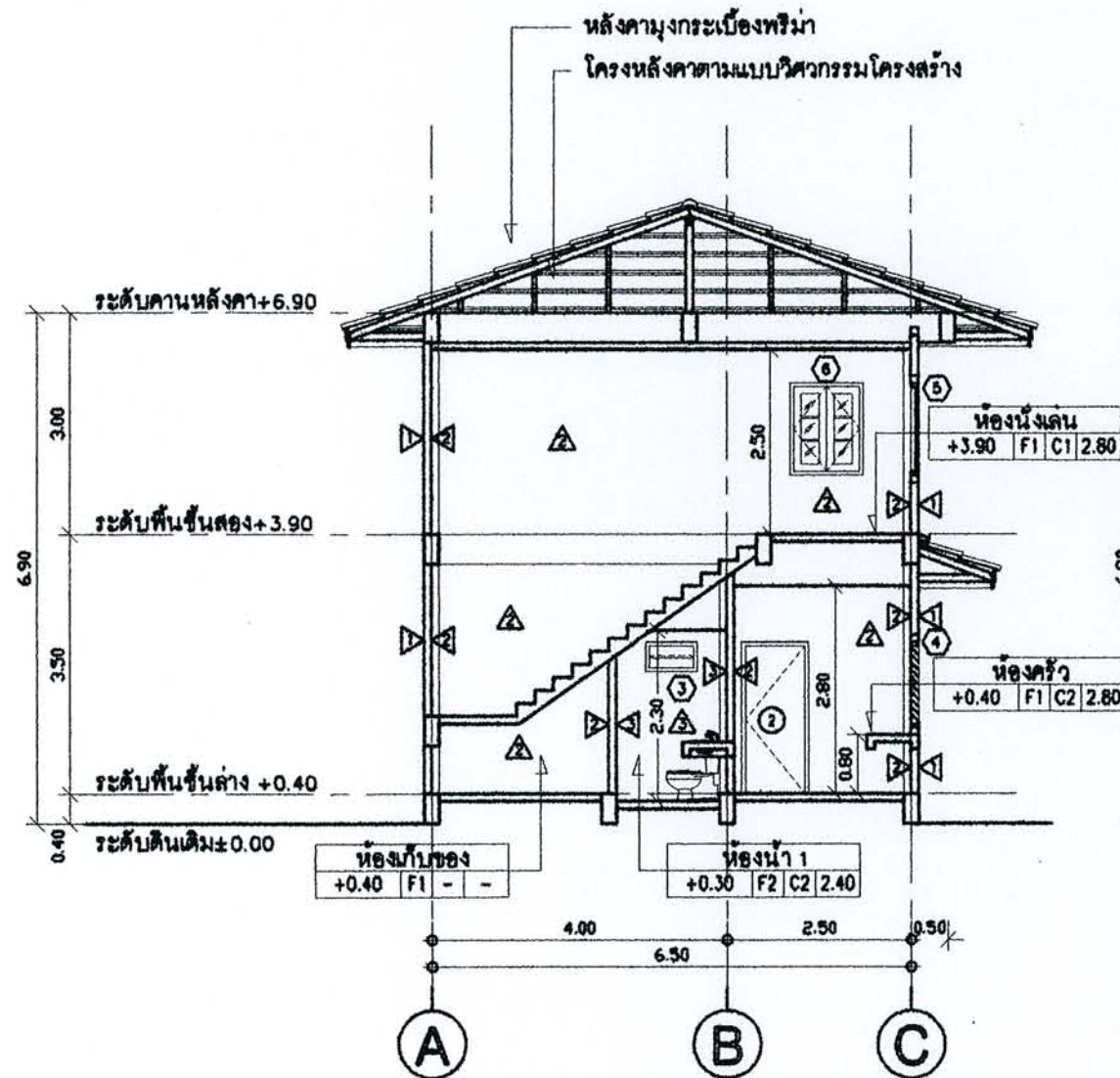
รูปตัด A มาตราส่วน 1:100
