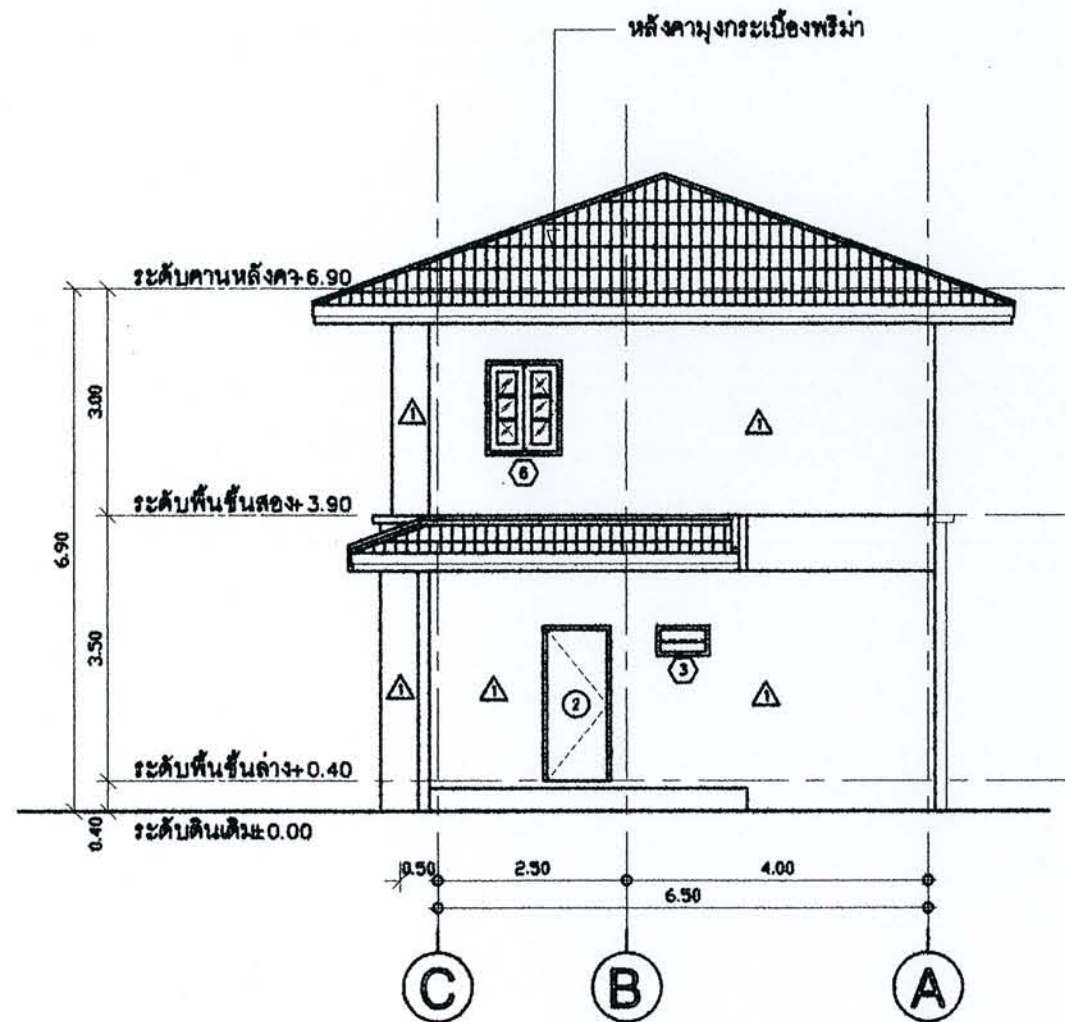
รูปด้าน 3
