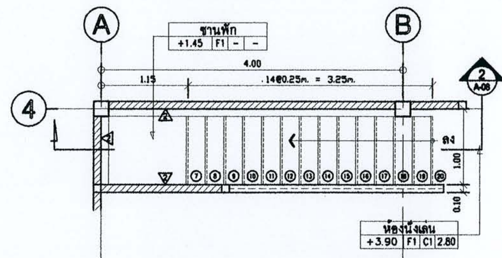
แปลนขยาย ST-2 ชั้นที่สอง มาตราส่วน 1:50
