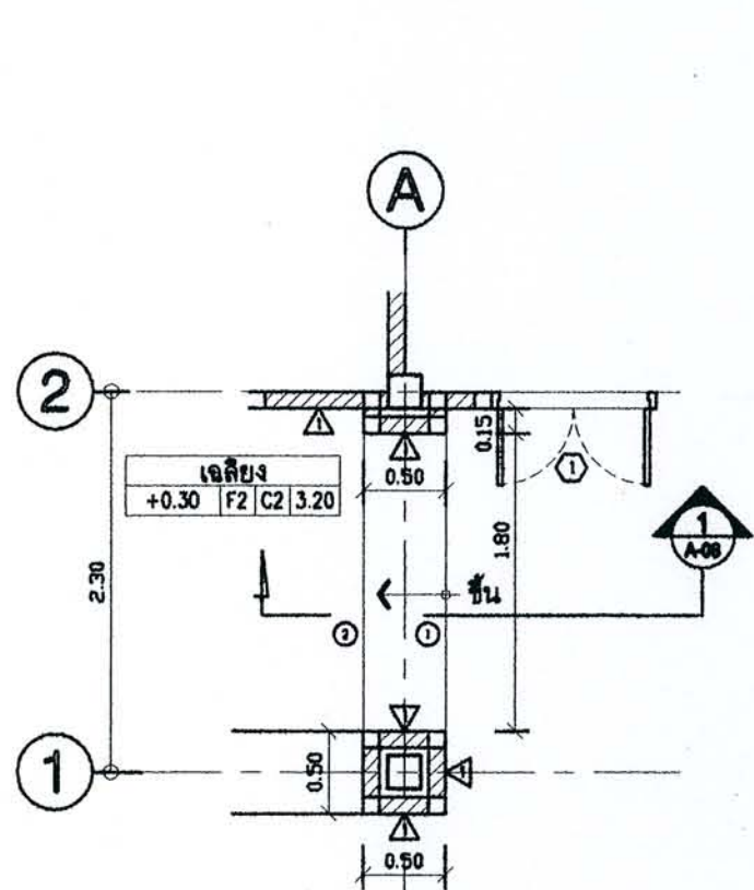
แปลนขยาย ST-1 มาตราส่วน 1:50
