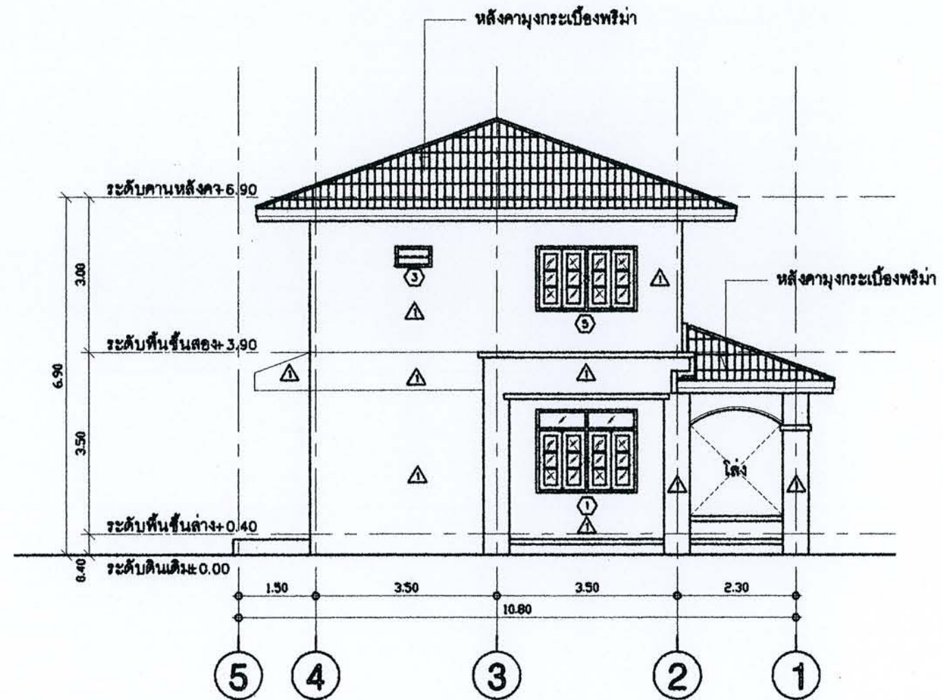
รูปด้าน 4
