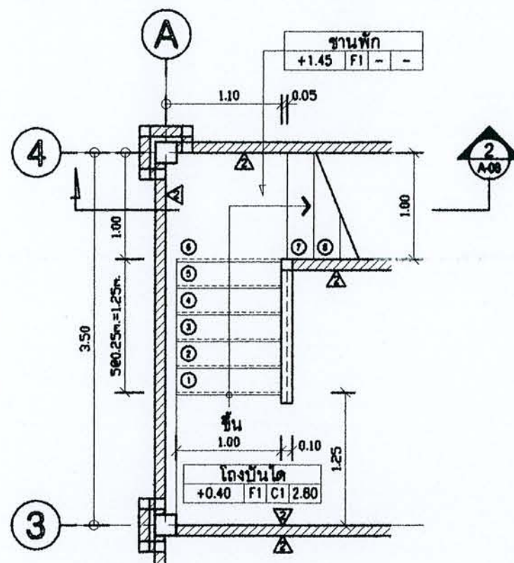
แปลนขยาย ST-2 ชั้นล่าง มาตราส่วน 1:50
