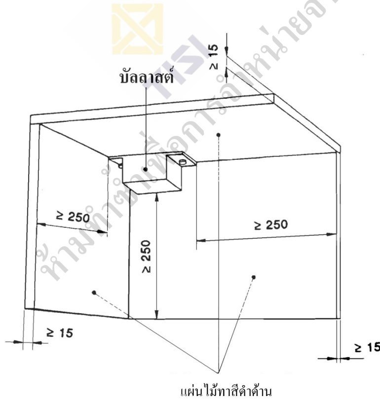
รูปที่ ๑.1 กล่องทดสอบสำหรับทดสอบการเกิดความร้อนของพลาสติก
