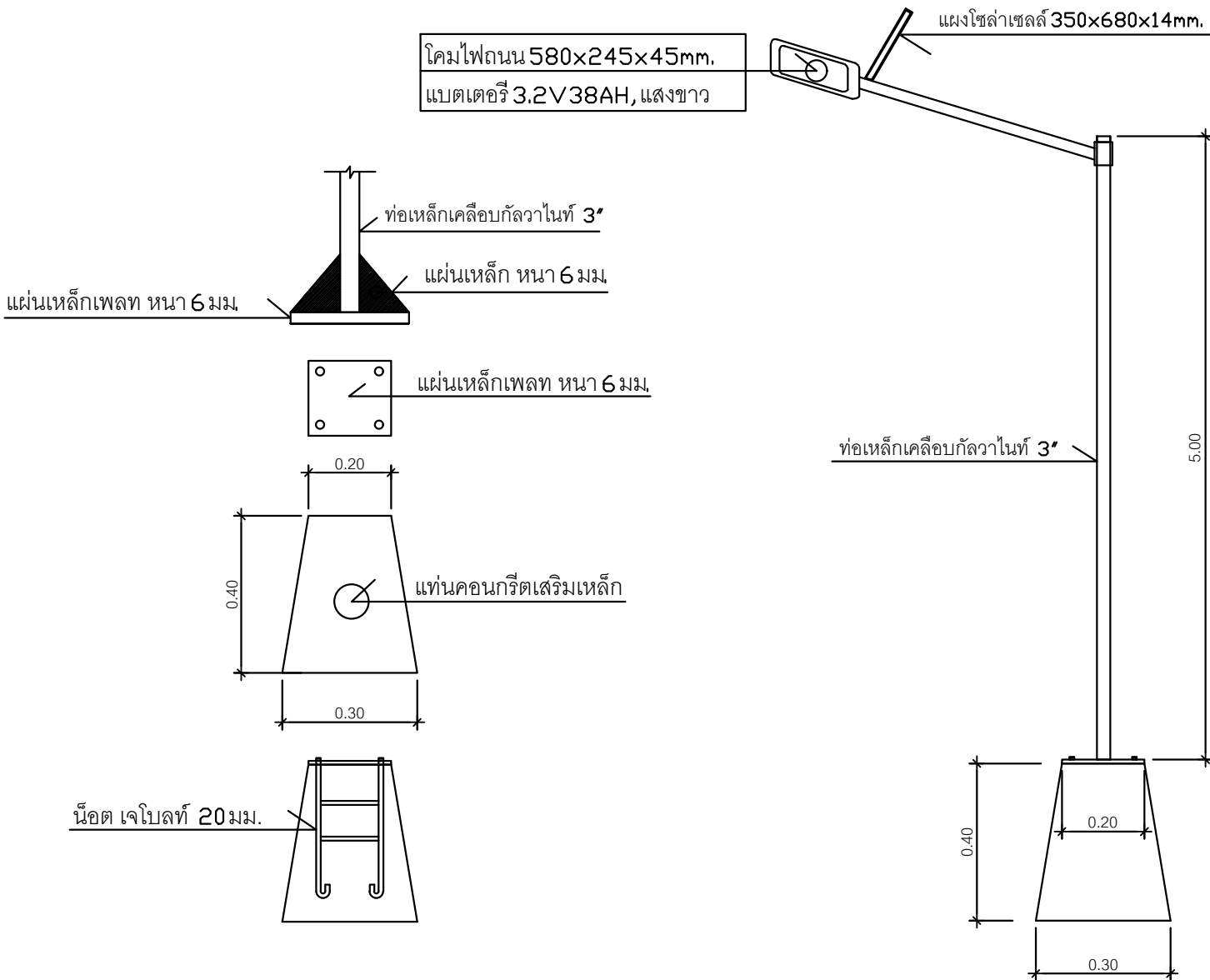
แบบไฟฟ้าพลังงานแสงอาทิตย์ (โซล่าเซลล์) No scale
