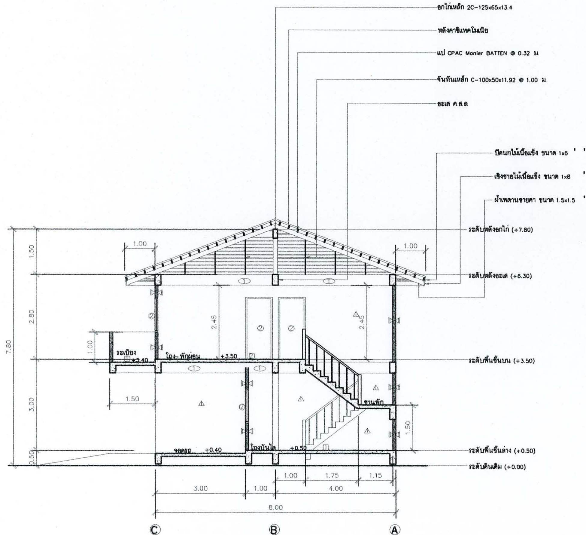
รูปตัด A-A ขนาดส่วน 1:75
