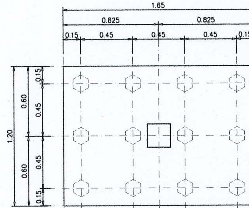
F-4 PLAN ขนาดตัว 1:20
