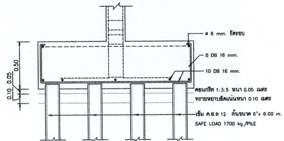
F-4 SECTION ขนาดตัว 1:20
