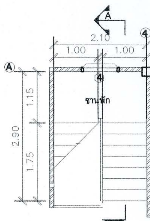
รูปขยายบันไดชั้นบน มาตราส่วน 1:50
