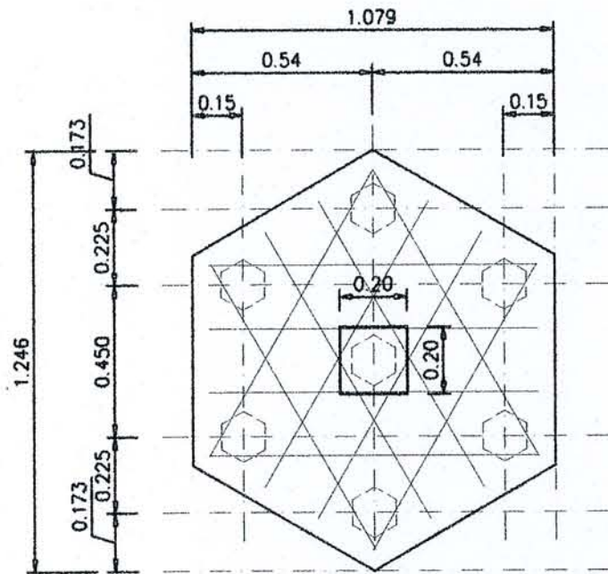
F-2 PLAN ขนาดตัว 1:20
