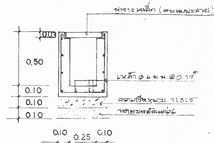
รูปตัด ข-ข 1:20
