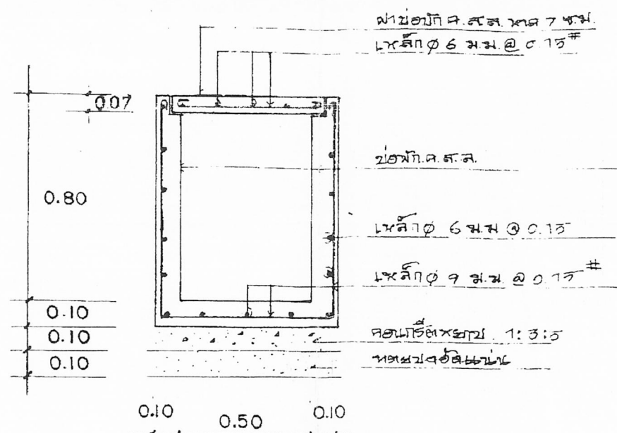
รูปตัด ก-ก 1:20
