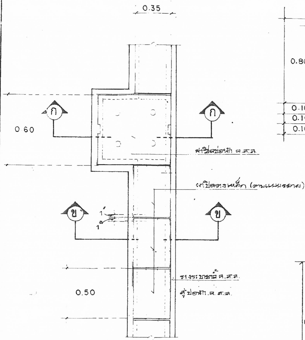
แบบร่างระบายน้ำ 1:20
