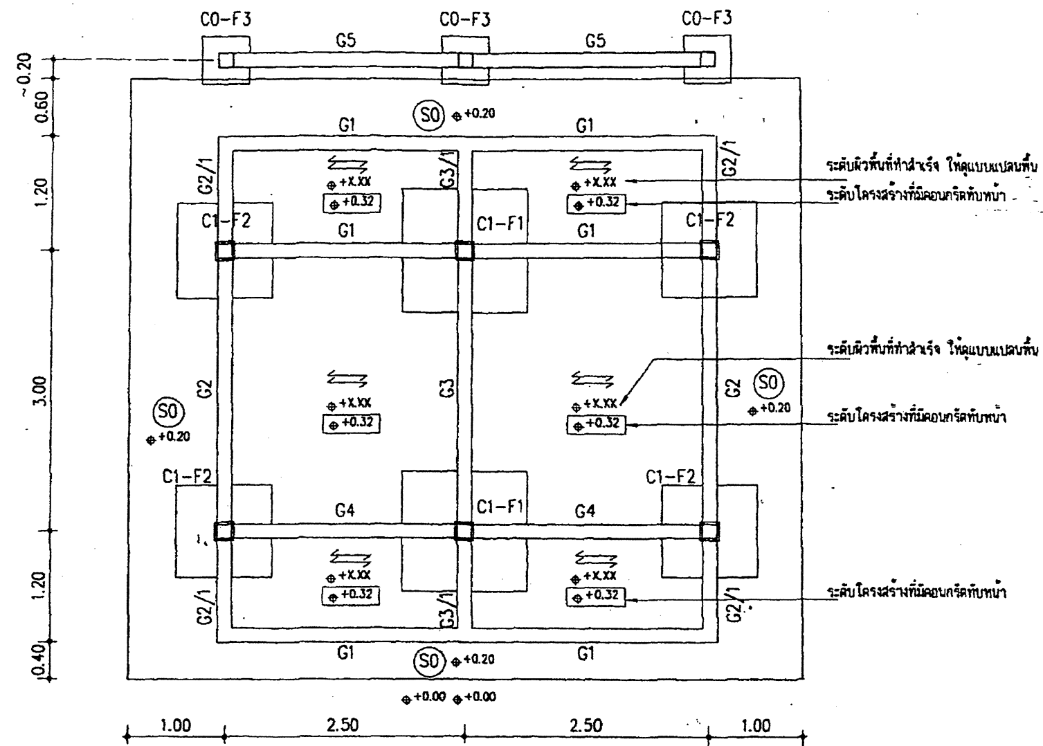
แปลนฐานรากและคานคอดิน มาตราส่วน 1:50
