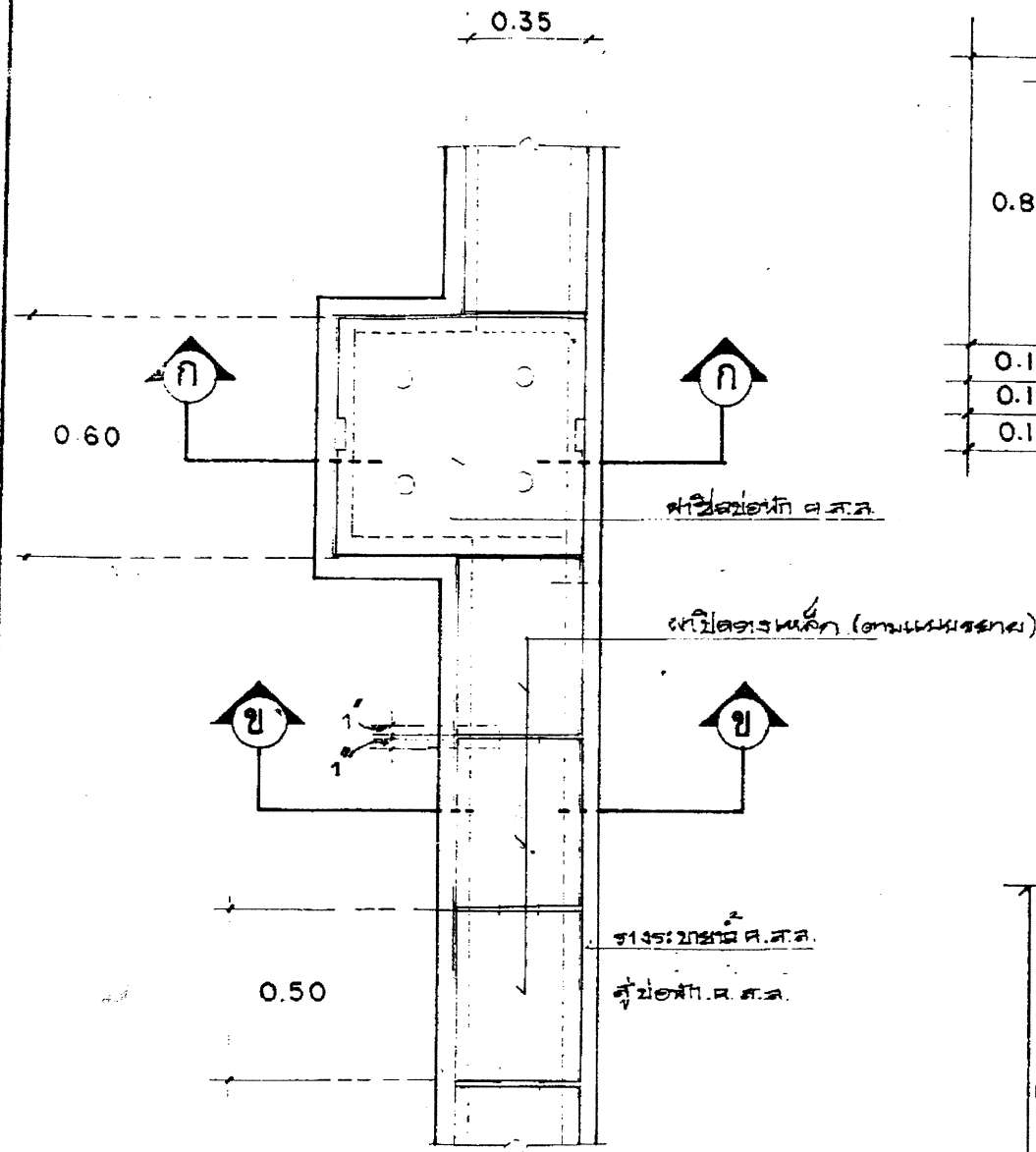
แปลนระบายน้ำ 1:20
