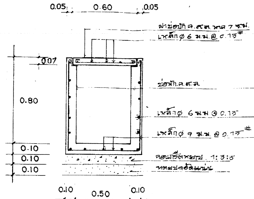
รูปตัด ก-ก 1:20
