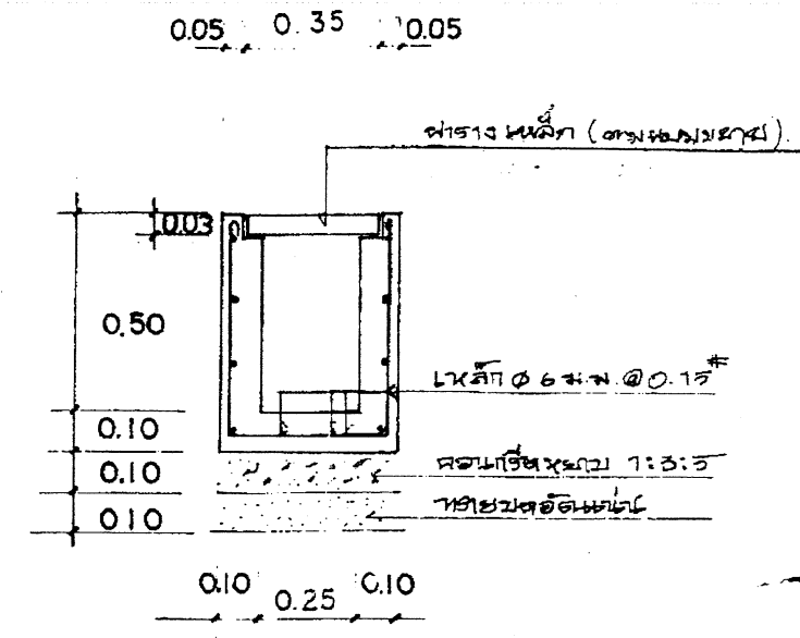
รูปตัด ข-ข 1:20
