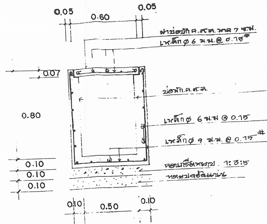
รูปตัด ก-ก 1:20
