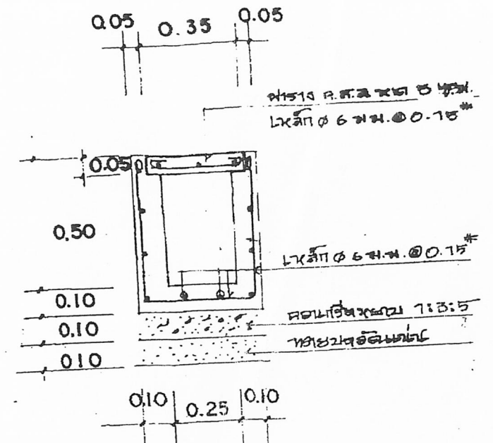
รูปตัด ข-ข 1:20
