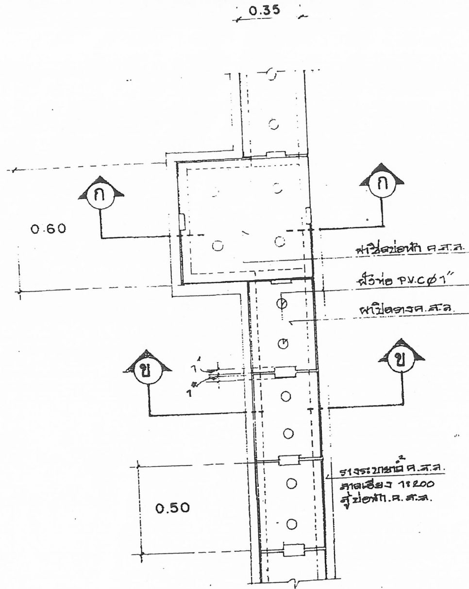
แปลนวางระบายน้ำเปิด 1:20
