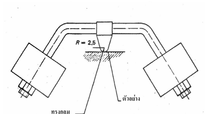
รูปที่ 25 เครื่องสำร็จทดสอบแรงกดด้วยลูกเหล็กกลม
