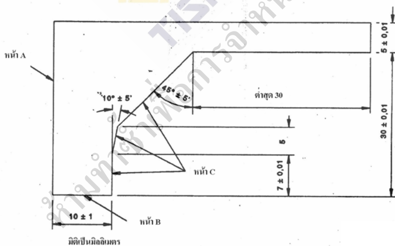
รูปที่ 20 เกจ (ความหนา: ประมาณ 2 มิลลิเมตร) สำหรับการทดสอบ
