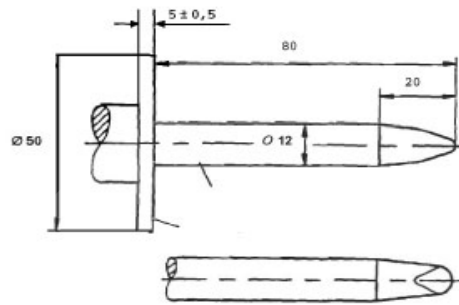
รูปที่ 9 น๊อตสอบแบบตรงไม่มีข้อ
