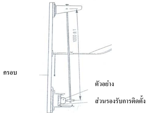
รูปที่ 15 เครื่องสำร็จทดสอบการกระแทก (ข้อ 20.1)
