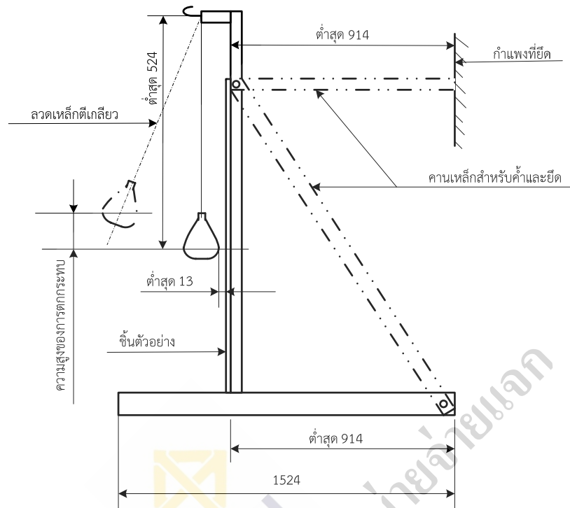
รูปที่ 10 การทดสอบความทนแรงกระแทกด้วยอุปกรณ์ (ข้อ 9.9.1 ข้อ 9.9.1.1 และข้อ 9.9.3)
