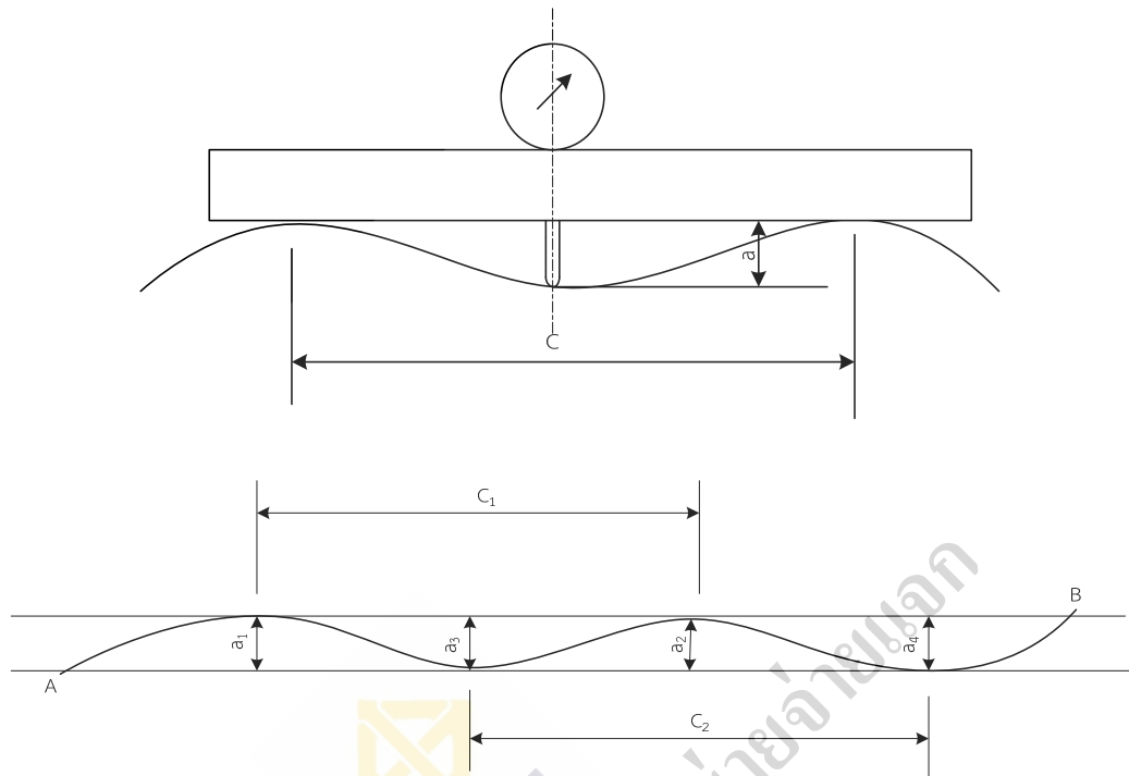
รูปที่ 8 การวัดความโค้งสำหรับโค้งแบบคลื่น (ข้อ 9.5.2.2 (2))
