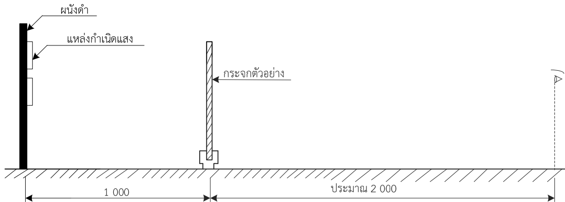
รูปที่ 2 การทดสอบหาดำหนี (ข้อ 9.2.2)
