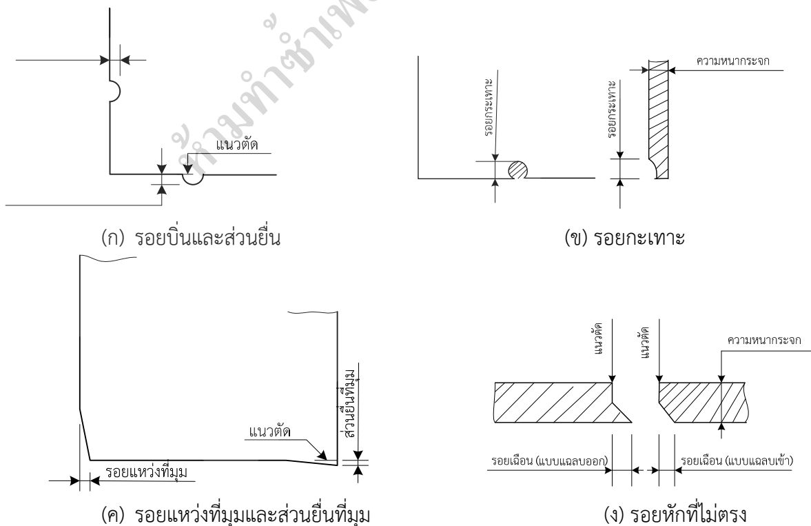
รูปที่ 3 ดำหนีที่ขอบ (ข้อ 9.3.2)
