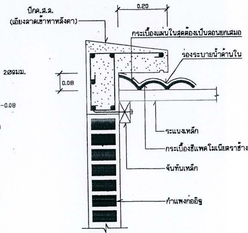
การทำปึก.ส.ล.ชนผนัง 1:10
