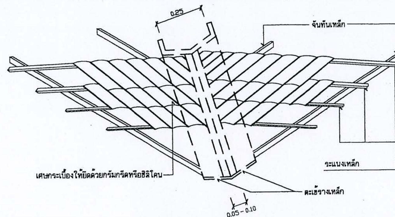
แบบขยายการทำตะเข้ราง 1:10
