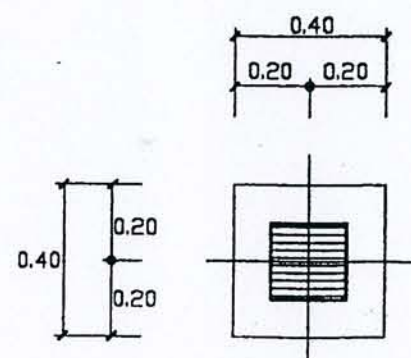
PLAN F1
