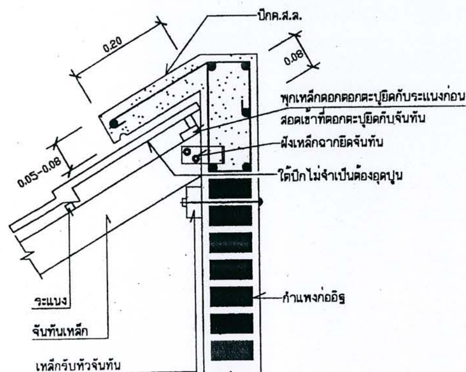
การทำปึก.ส.ล.ชนผนัง 1:10
