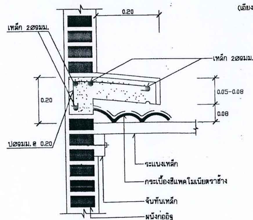
การทำปึก.ส.ล.ชนผนัง 1:10
