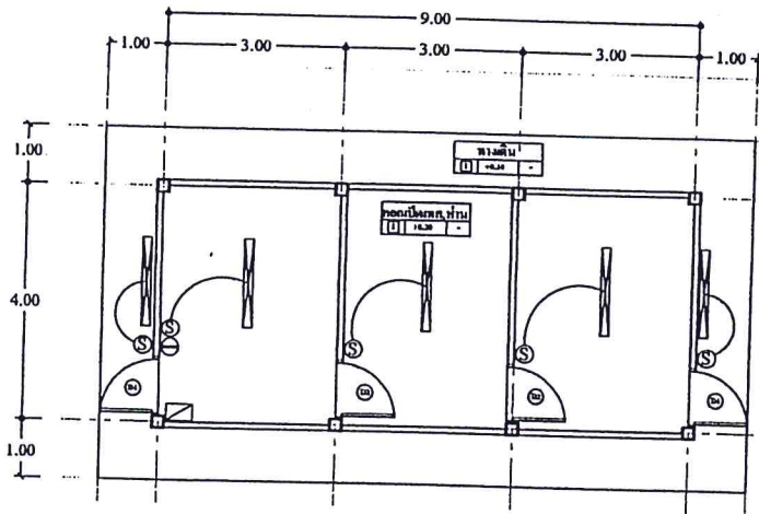
แปลนไฟฟ้า
