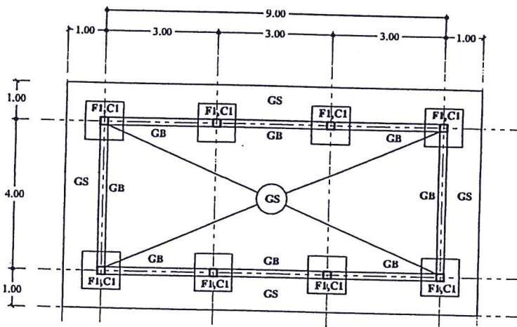
แปลนโครงสร้างฐานราก, เสา, คาน
