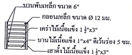
แบบขยายประตู D2
