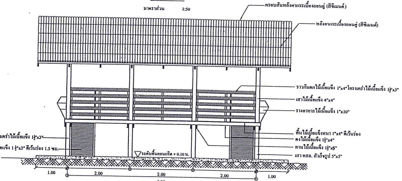
รูปด้านหลัง
