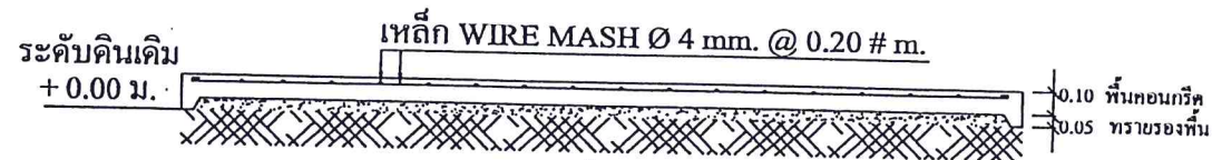
แบบขยายพื้นคอนกรีต
