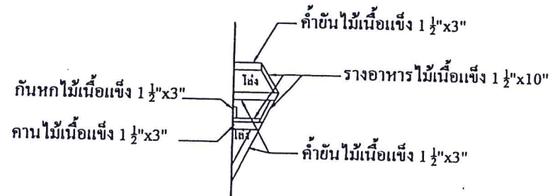
แบบขยายรางอาหาร
