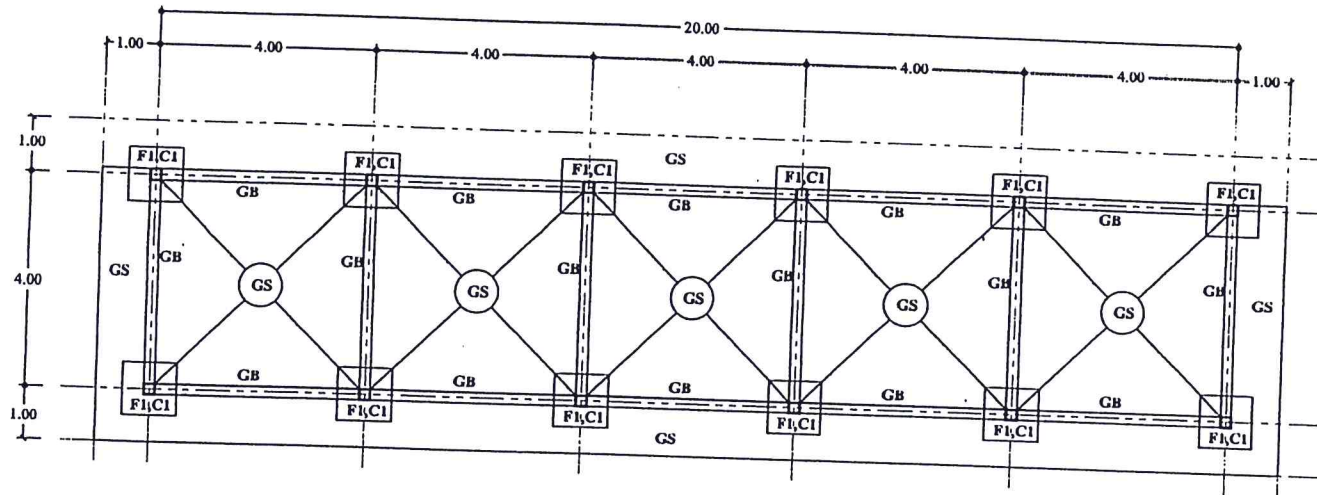
แปลนโครงสร้างฐานราก,เสา,คาน
