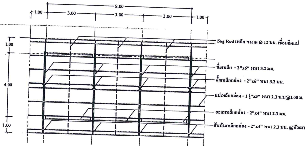
แปลนโครงสร้างคาน
