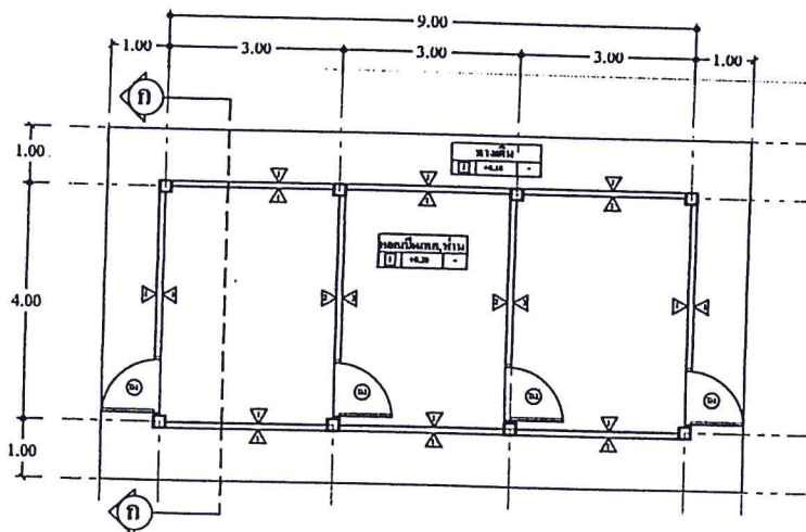
แปลนพื้น
