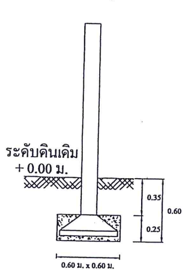
แบบขยายฐานราก มาตราส่วน 1:25
