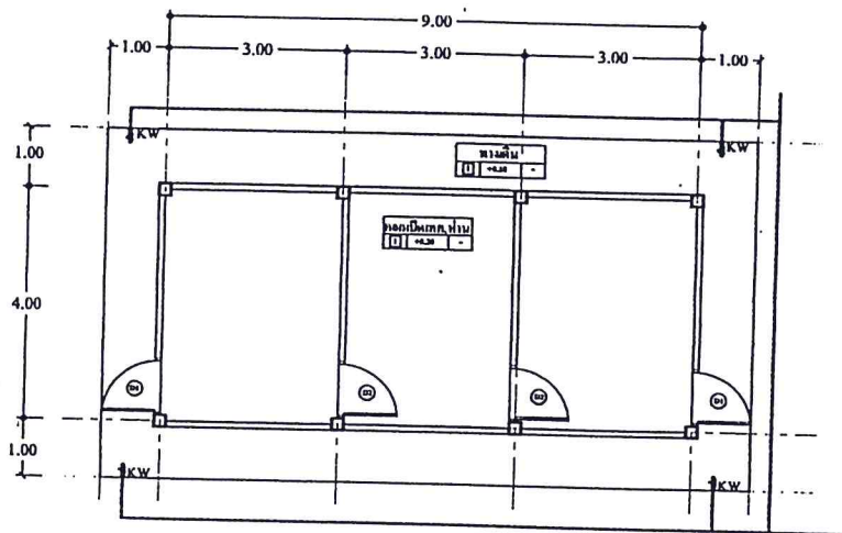
แปลนประปา
