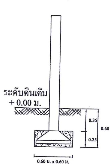
แบบขยายฐานราก
