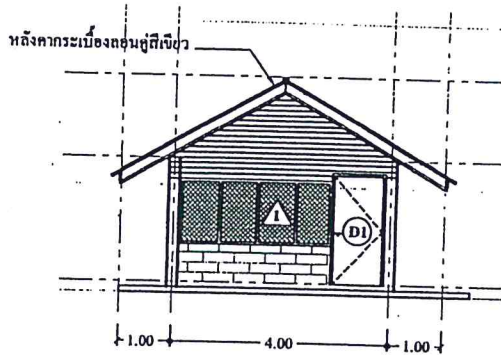
รูปด้าน หน้า - หลัง
