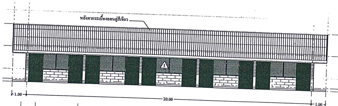
รูปด้าน หน้า
