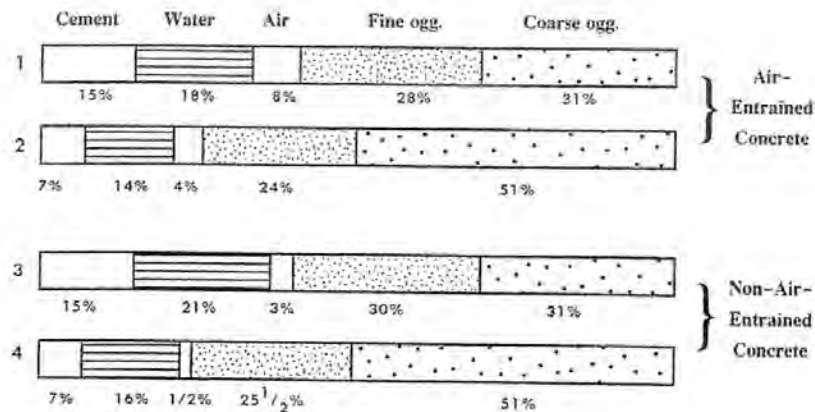
รูปที่ 1 ปริมาตรของส่วนผสมคอนกรีต ปริมาตรส่วนผสมที่ 1 และ 3 เป็นส่วนผสมแก่ปูนมีวัสดุผสมน้อย ส่วนปริมาตรส่วนผสมที่ 2 และ 4 เป็นส่วนผสมอ่อนปูนมีวัสดุผสมมาก
