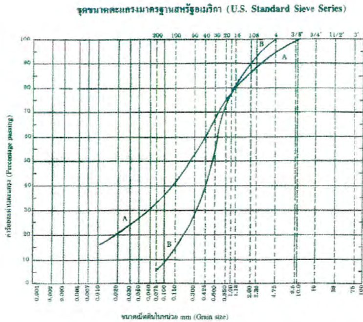
รูปที่ 1 กราฟชุดตะแกรงมาตรฐานสหรัฐอเมริกา (US Standard Sieve Series)
