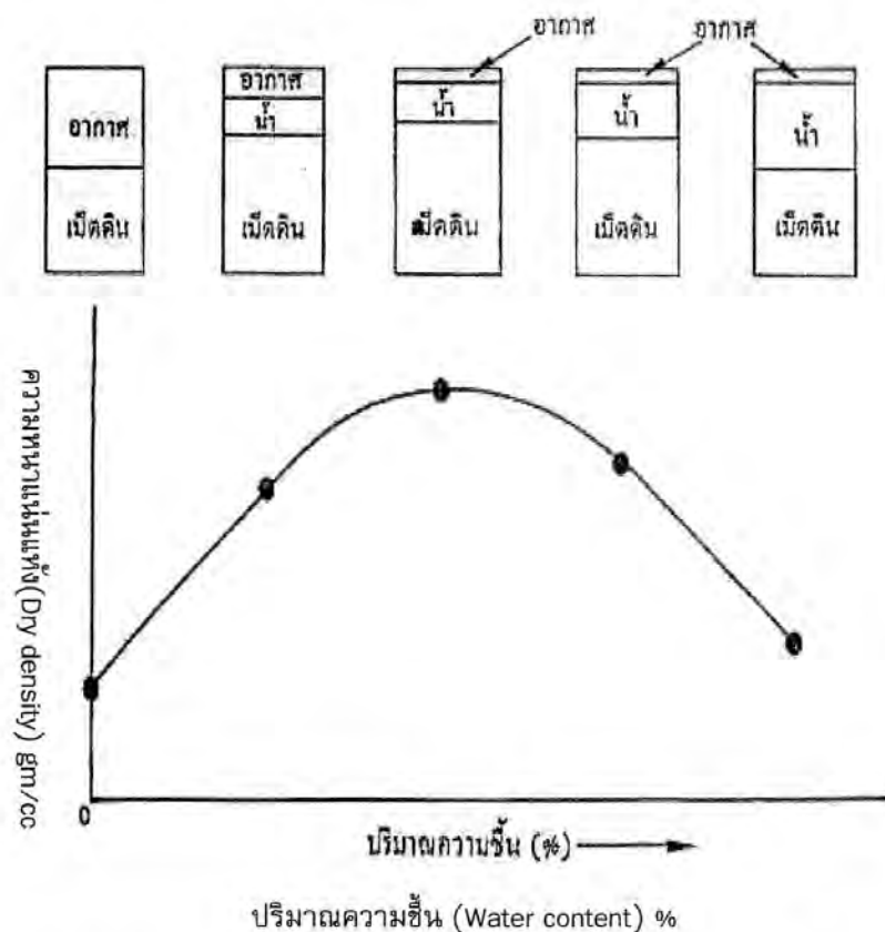
รูปที่ 20 กราฟแสดงความสัมพันธ์ระหว่างค่าความหนาแน่นแห้งและค่าปริมาณความชื้น
