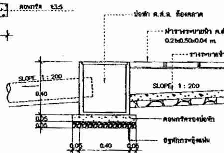
รูปตัดท่อระบายน้ำชนิดเปิดฝ้า
